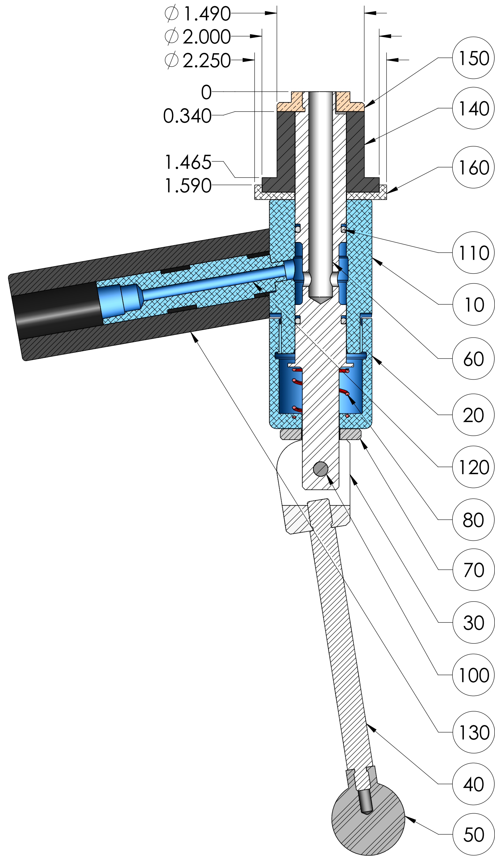
SECTION A-A
