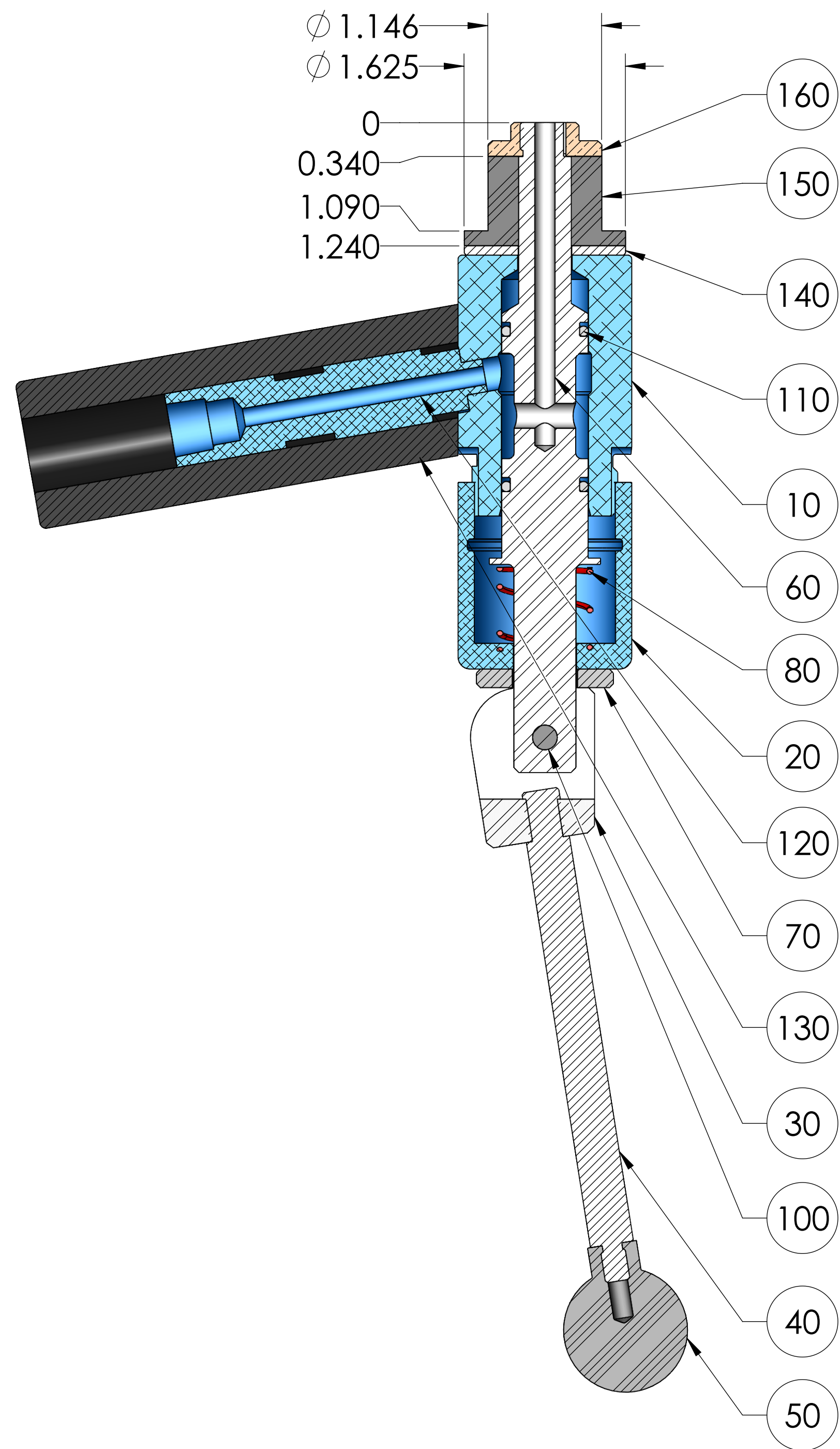
SECTION A-A
