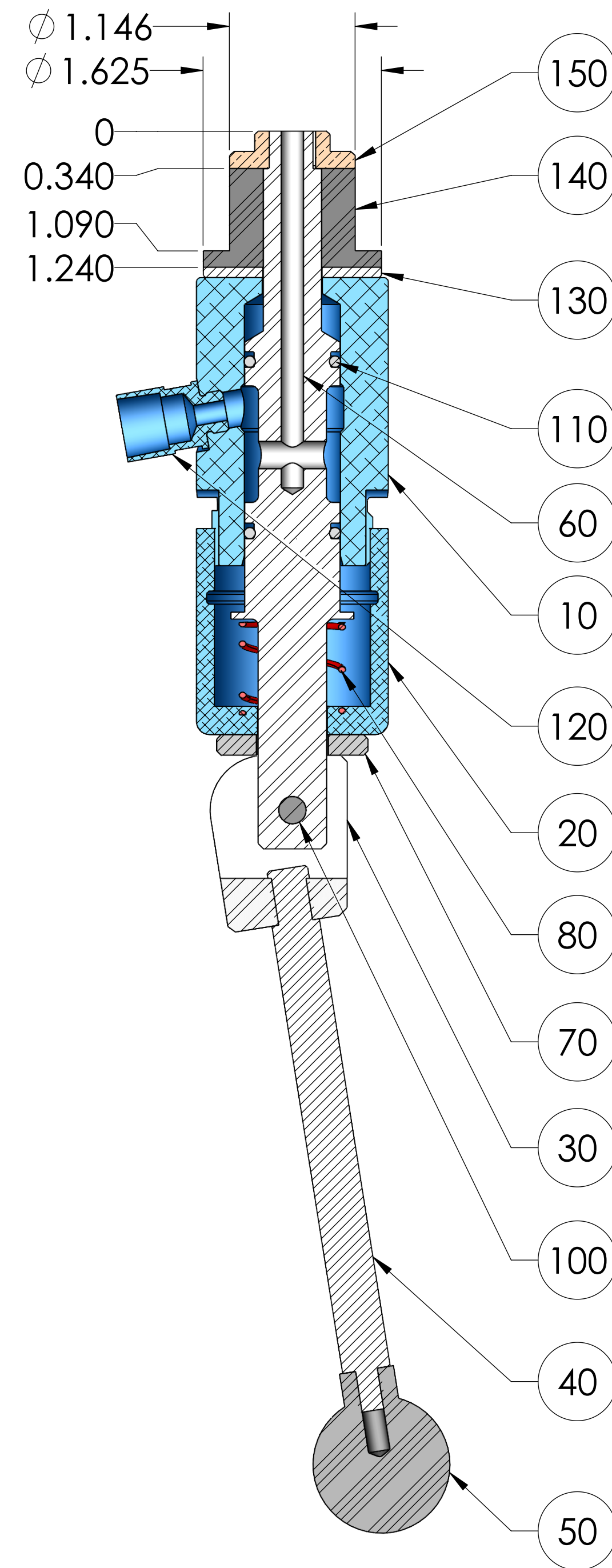
SECTION A-A
