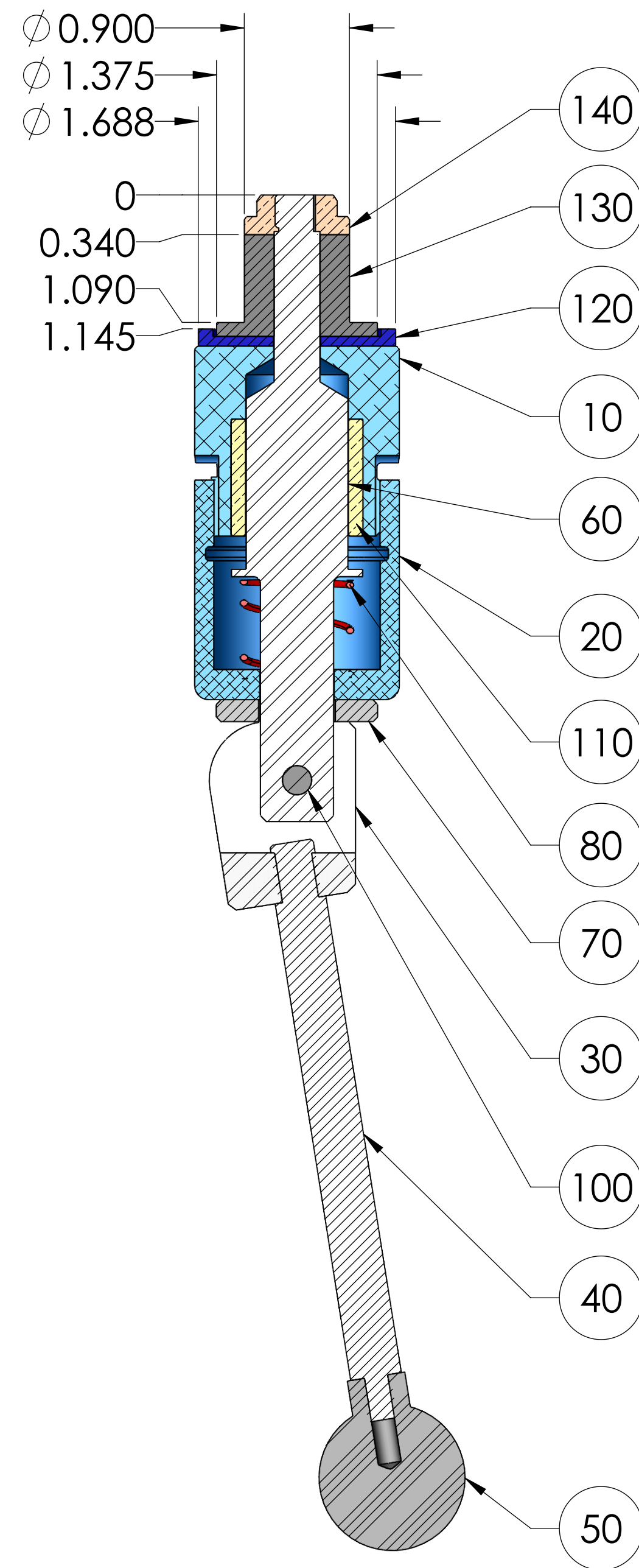
SECTION A-A
