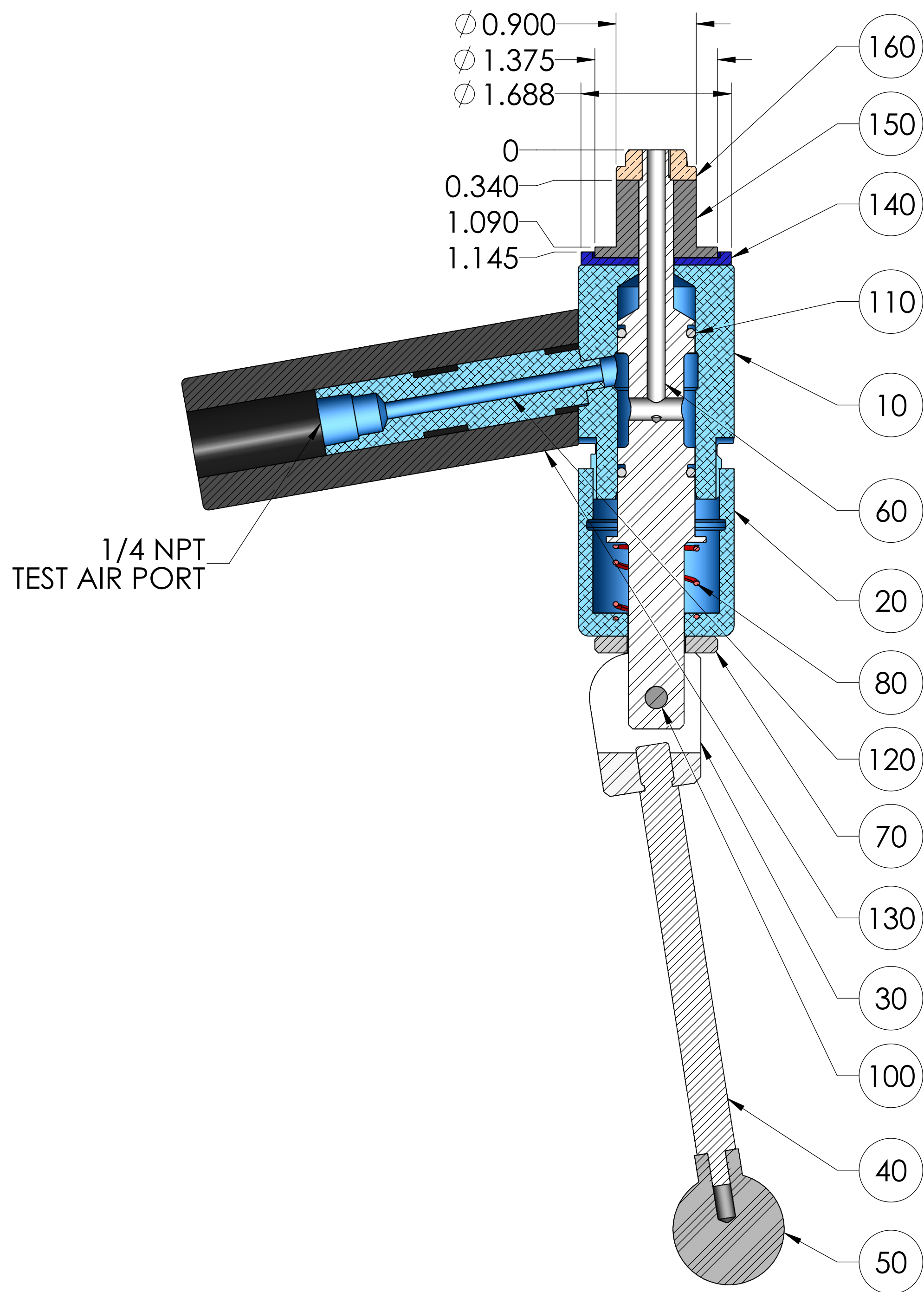
SECTION A-A
