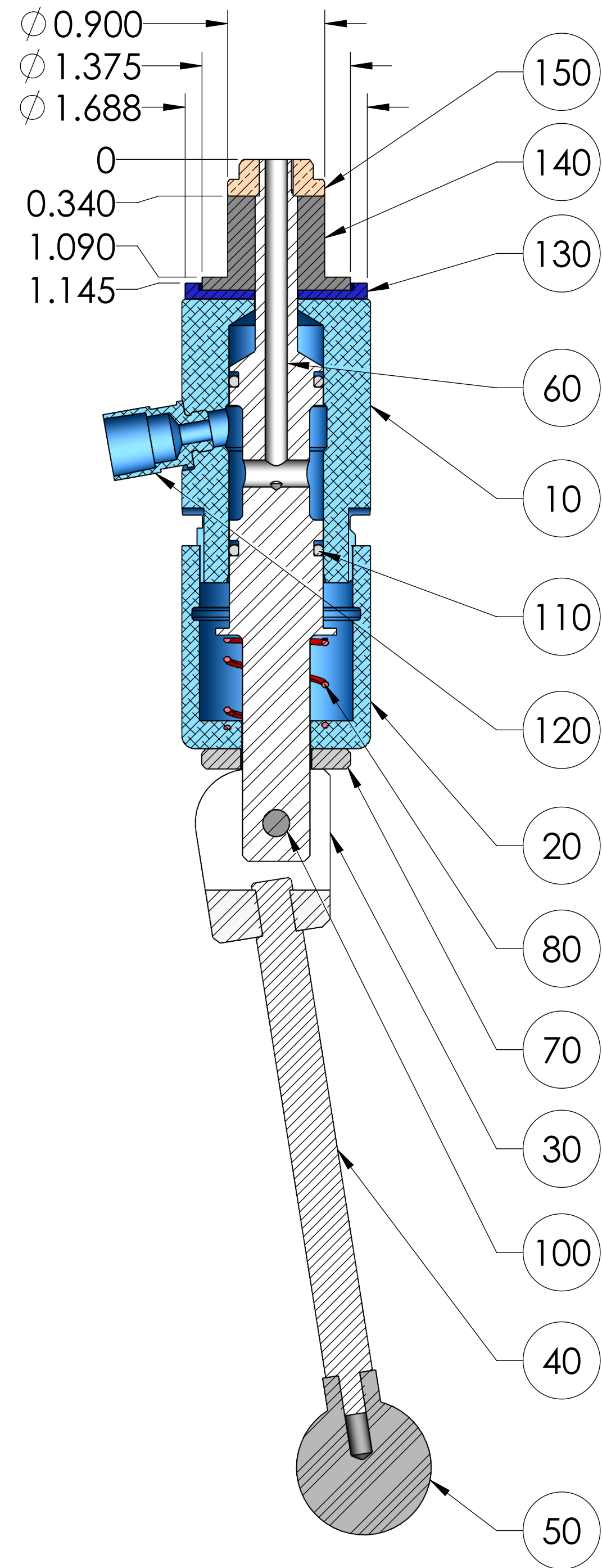
SECTION A-A
