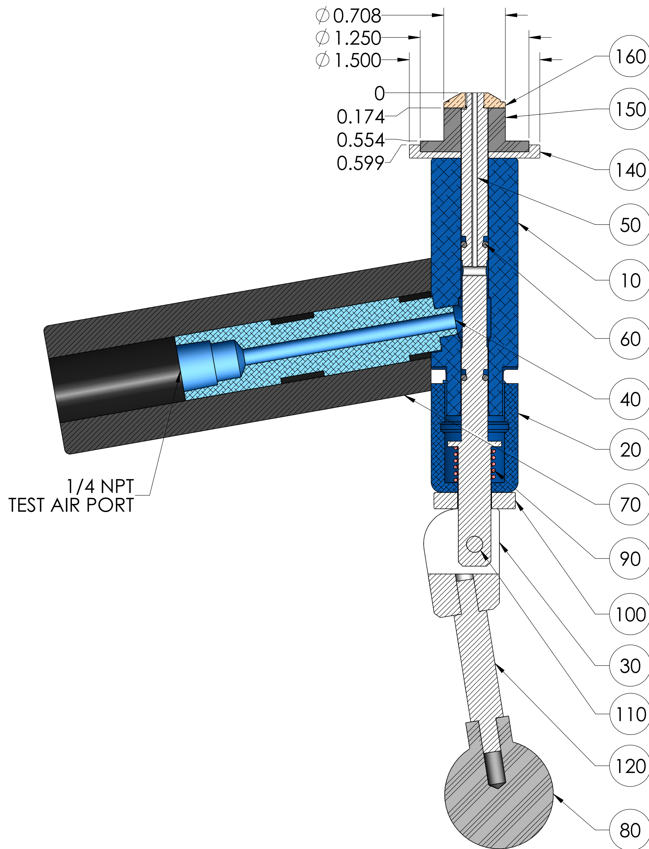
SECTION A-A SCALE 1.5 : 1
