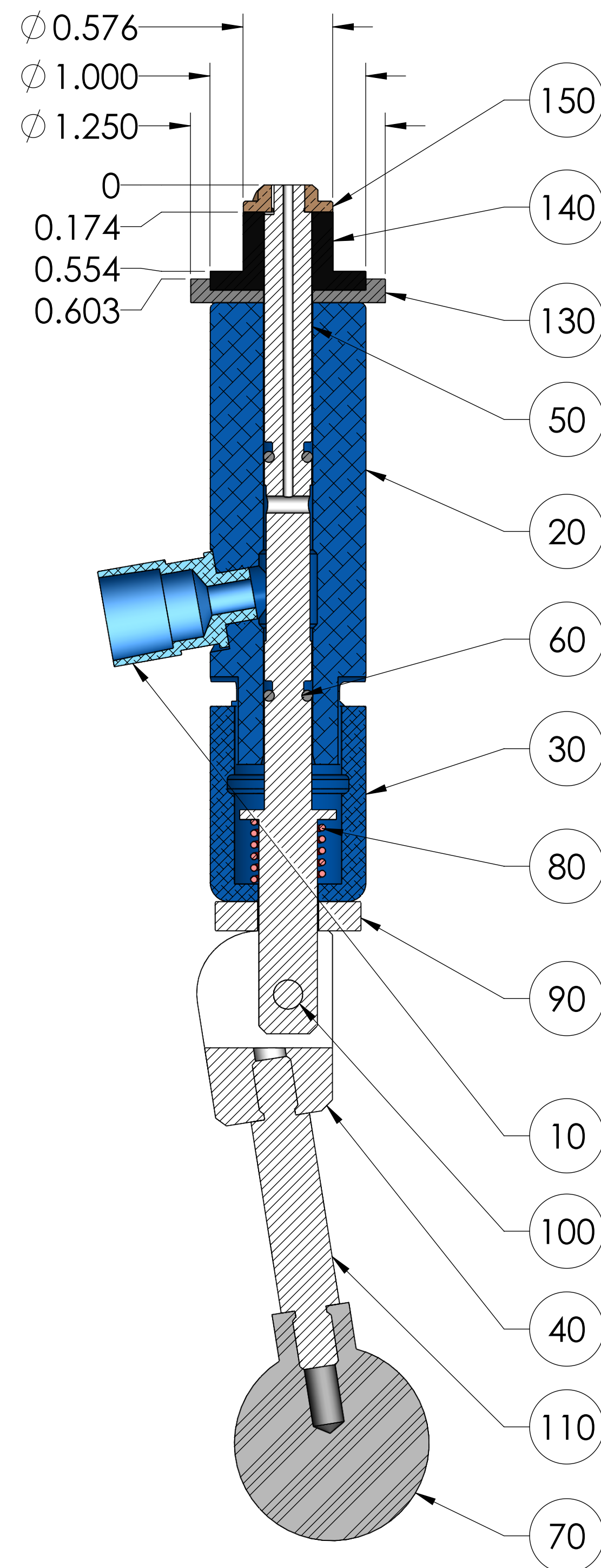
SECTION A-A SCALE 1.5 : 1
