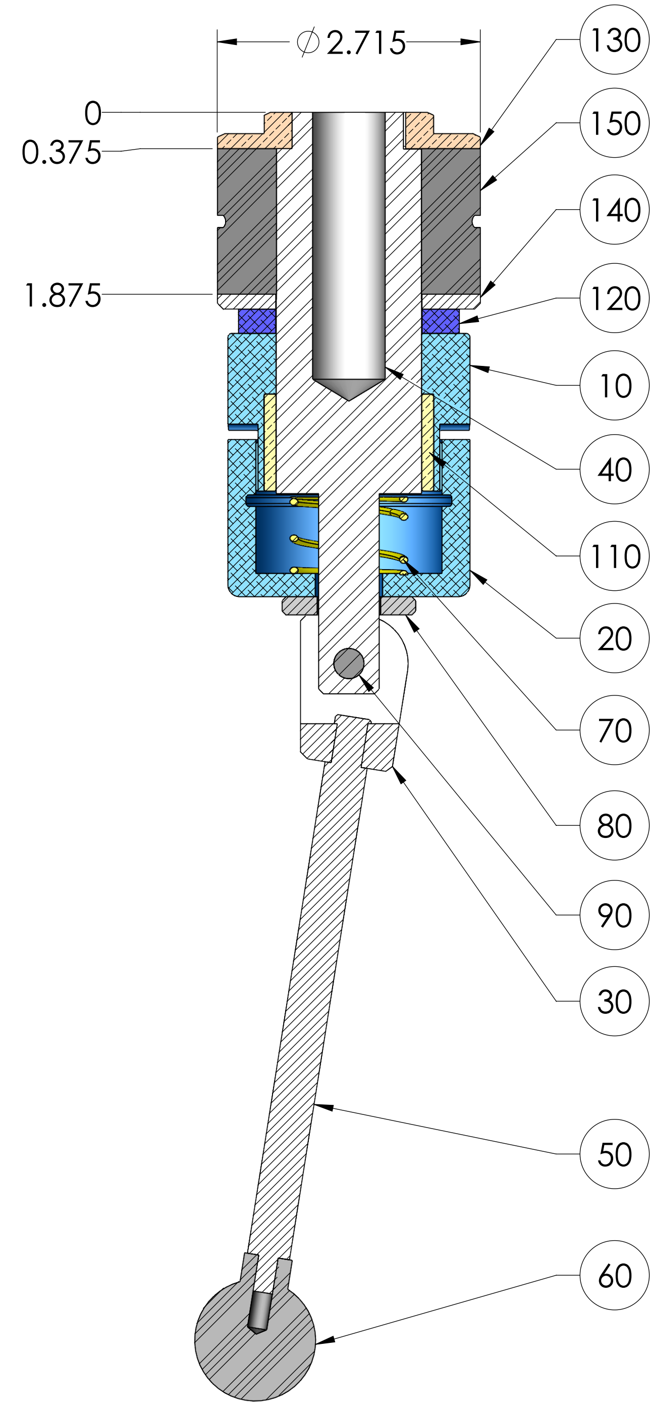
SECTION A-A SCALE 1 : 1
