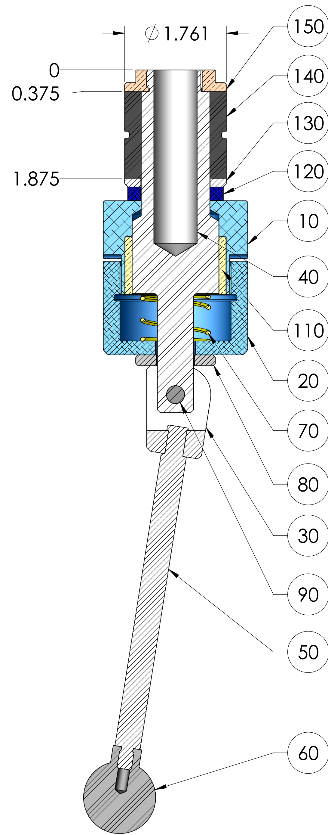
SECTION A-A SCALE 1 : 1
