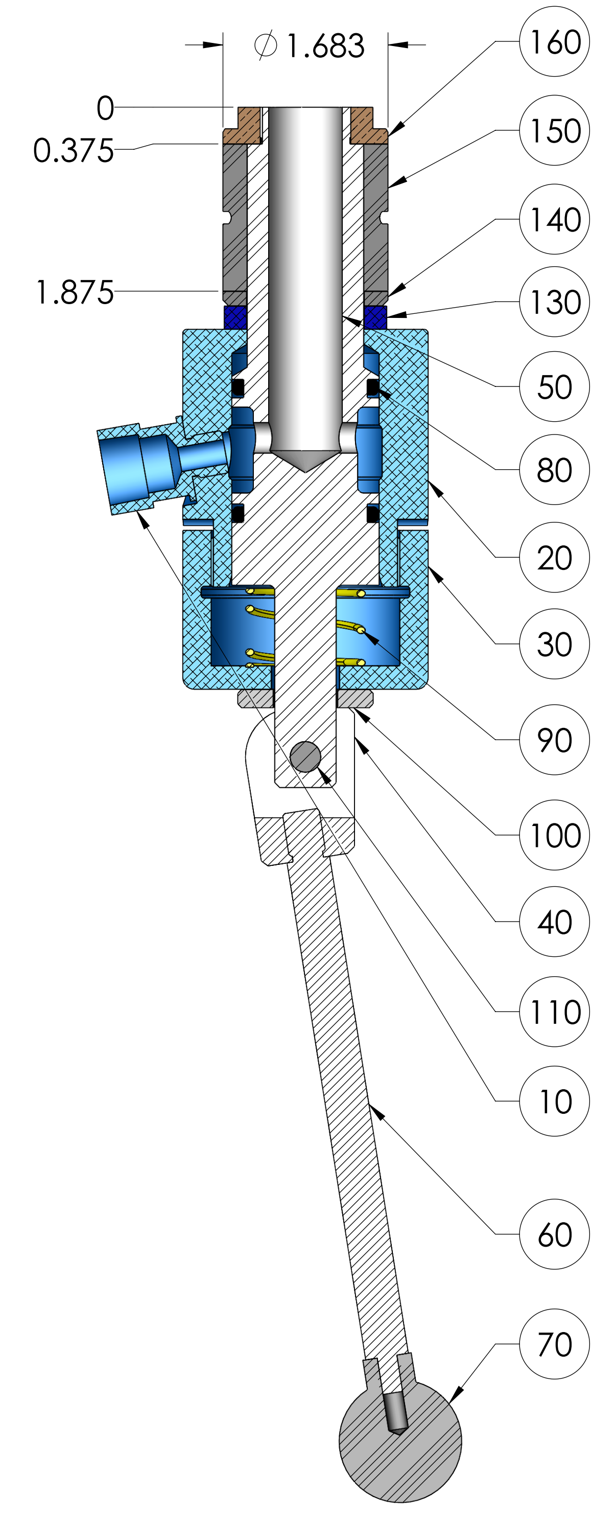
SECTION A-A SCALE 1 : 1
