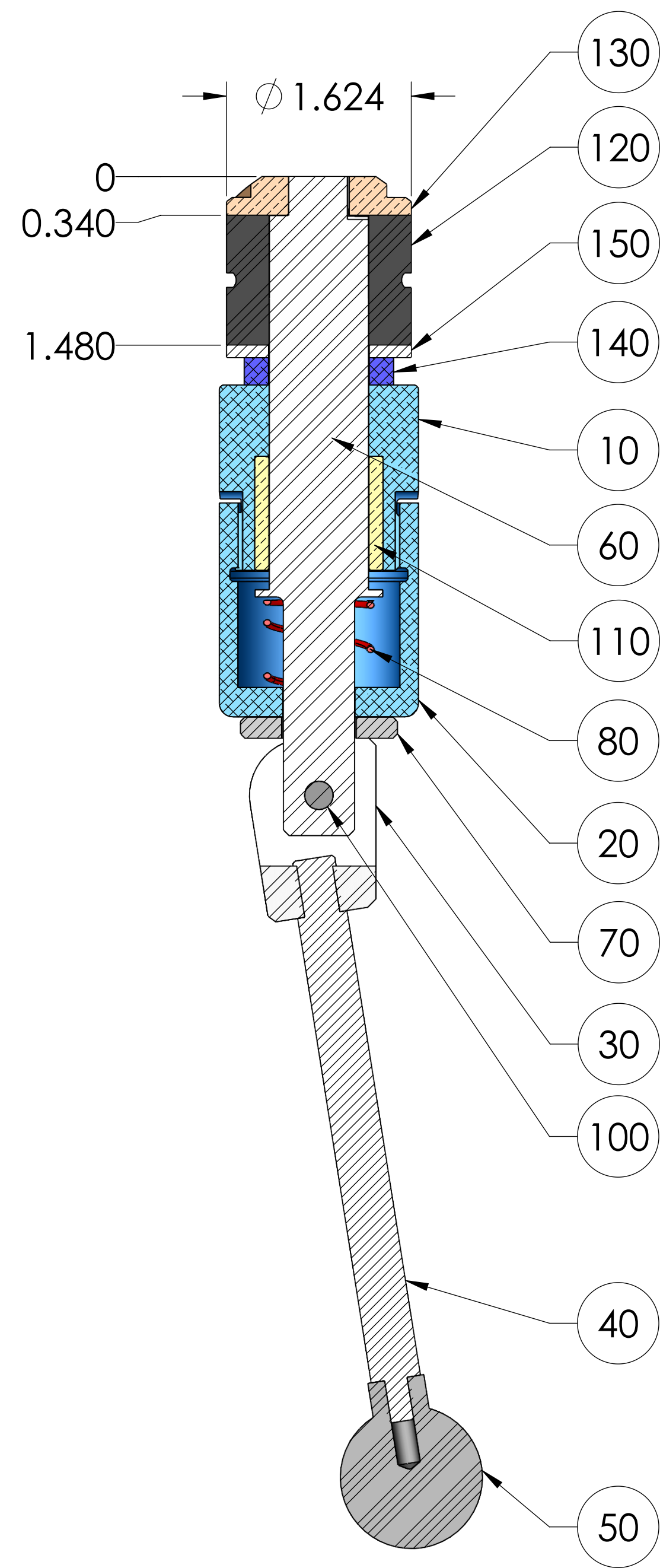
SECTION A-A
