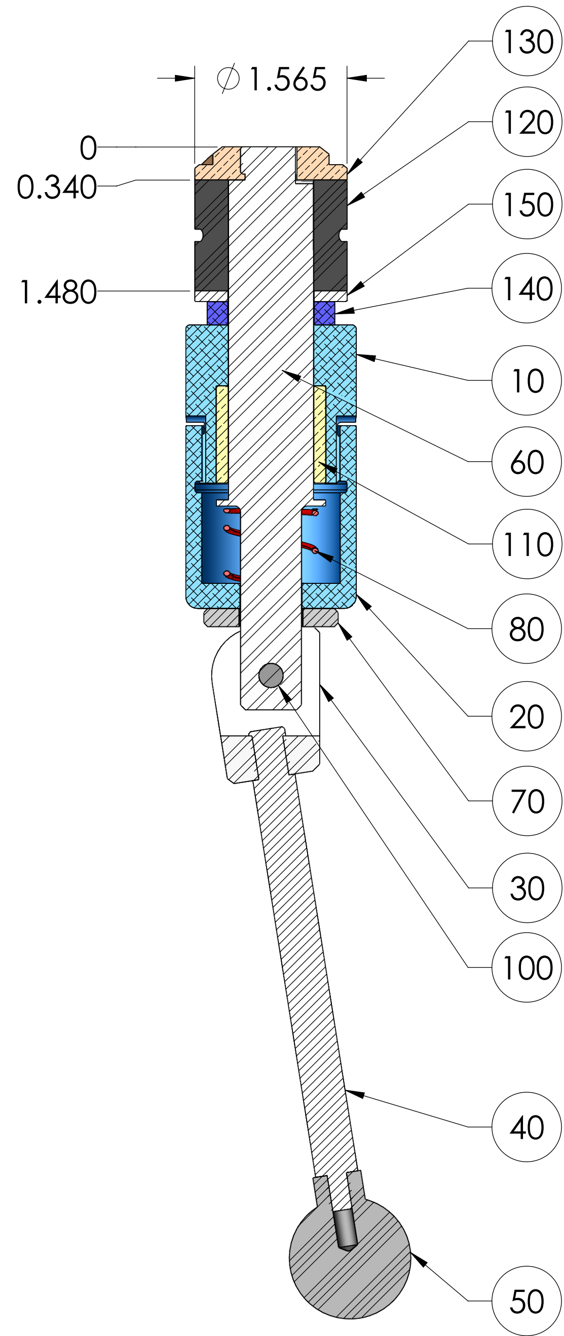
SECTION A-A
