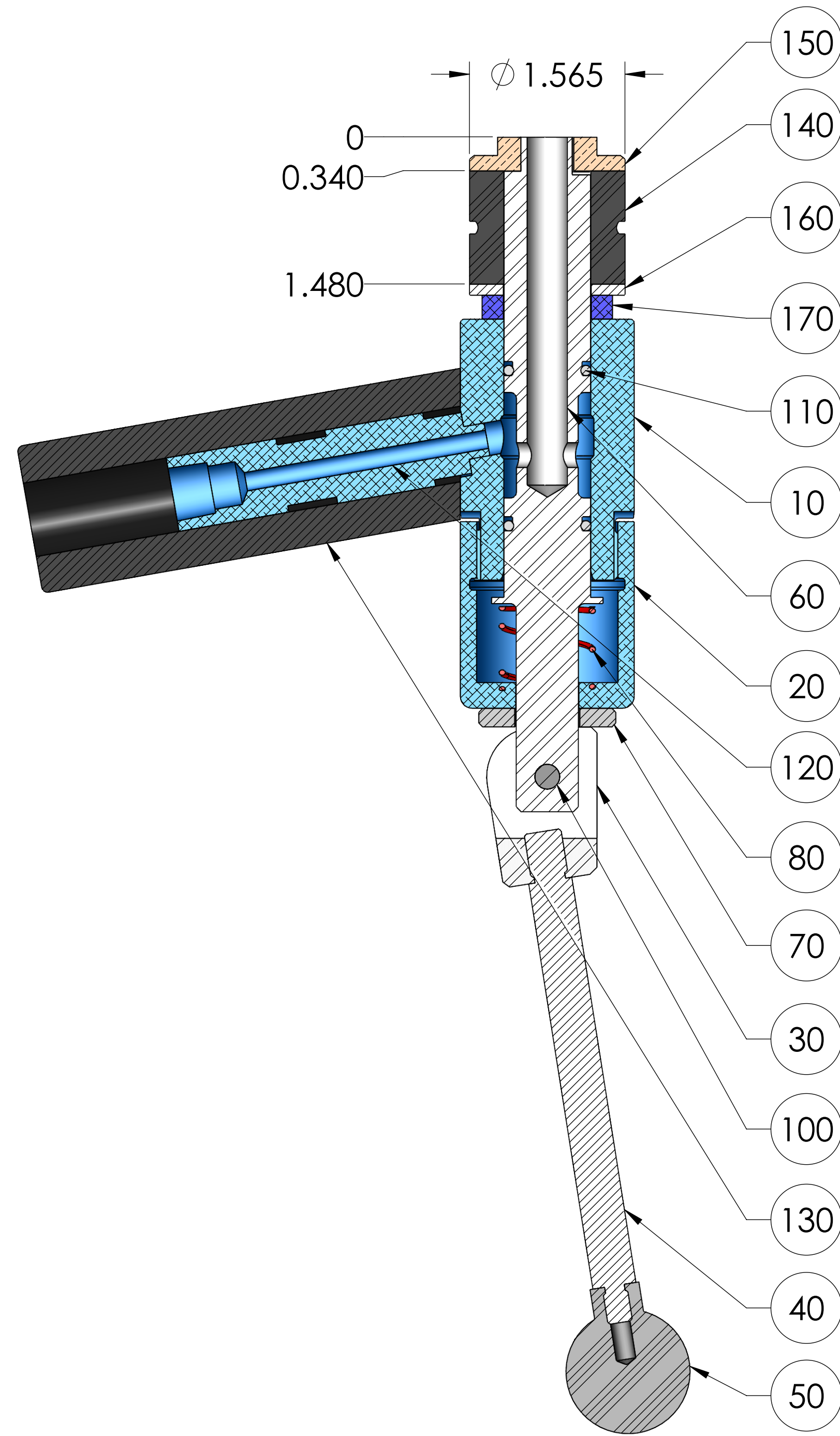
SECTION A-A
