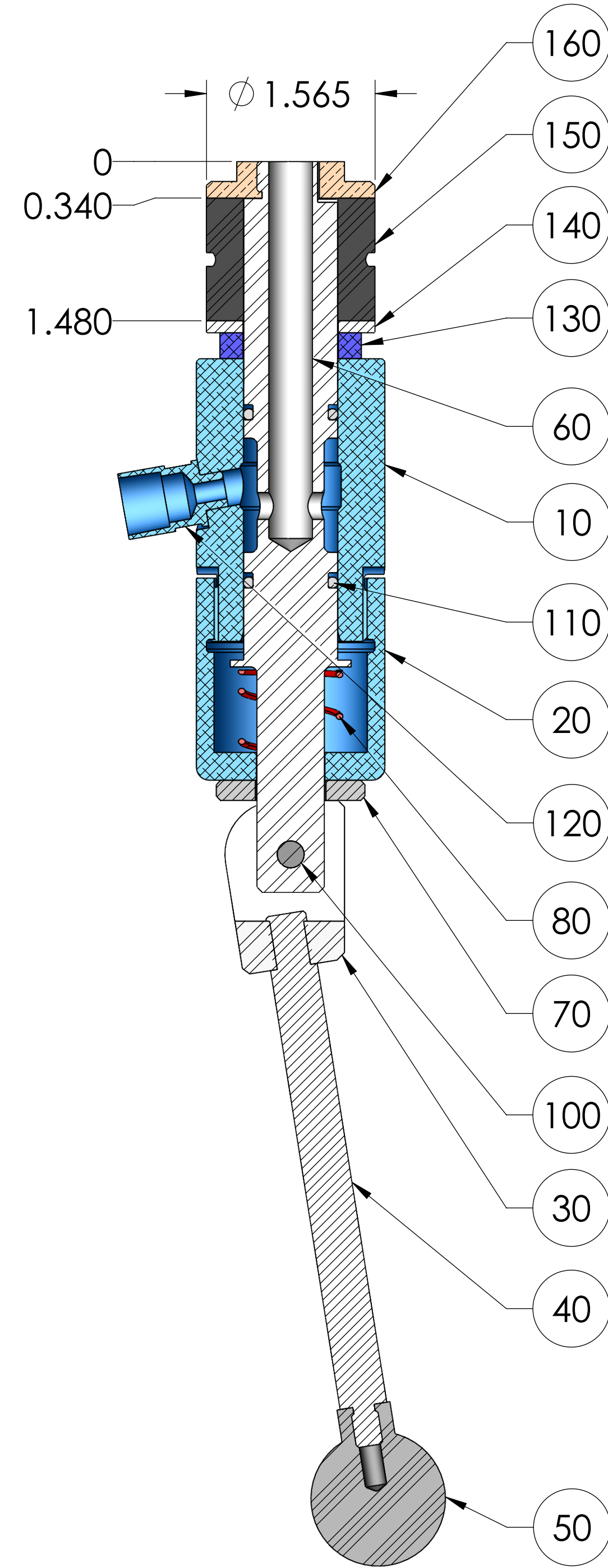
SECTION A-A
