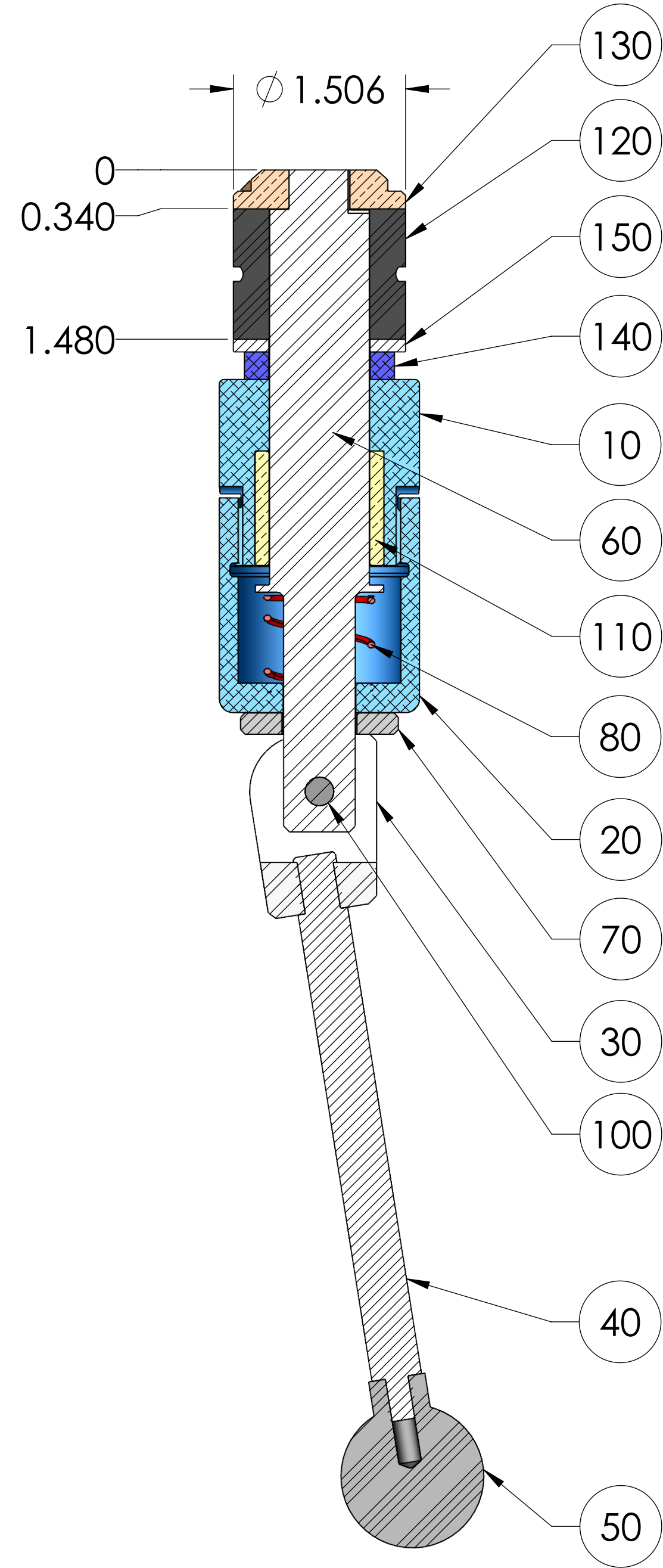
SECTION A-A
