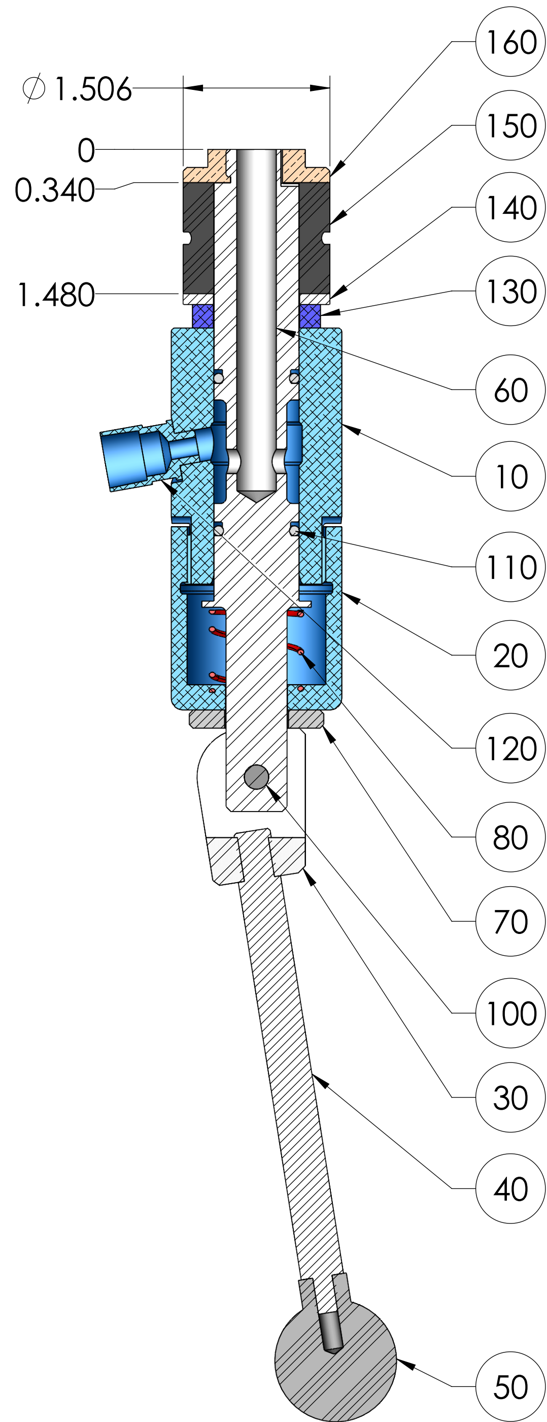
SECTION A-A
