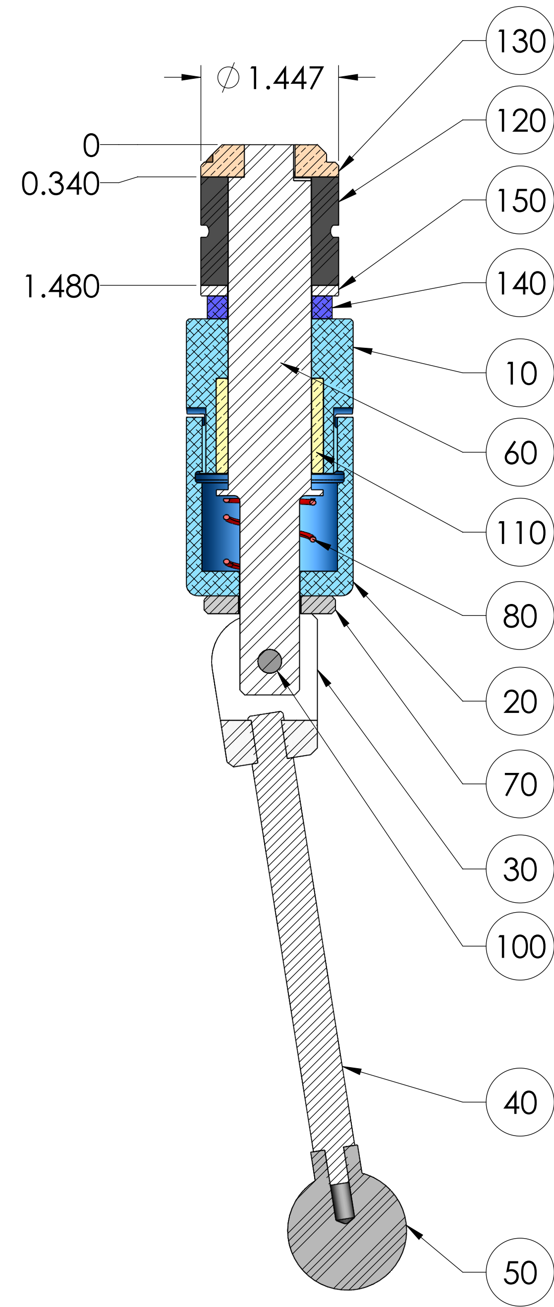
SECTION A-A
