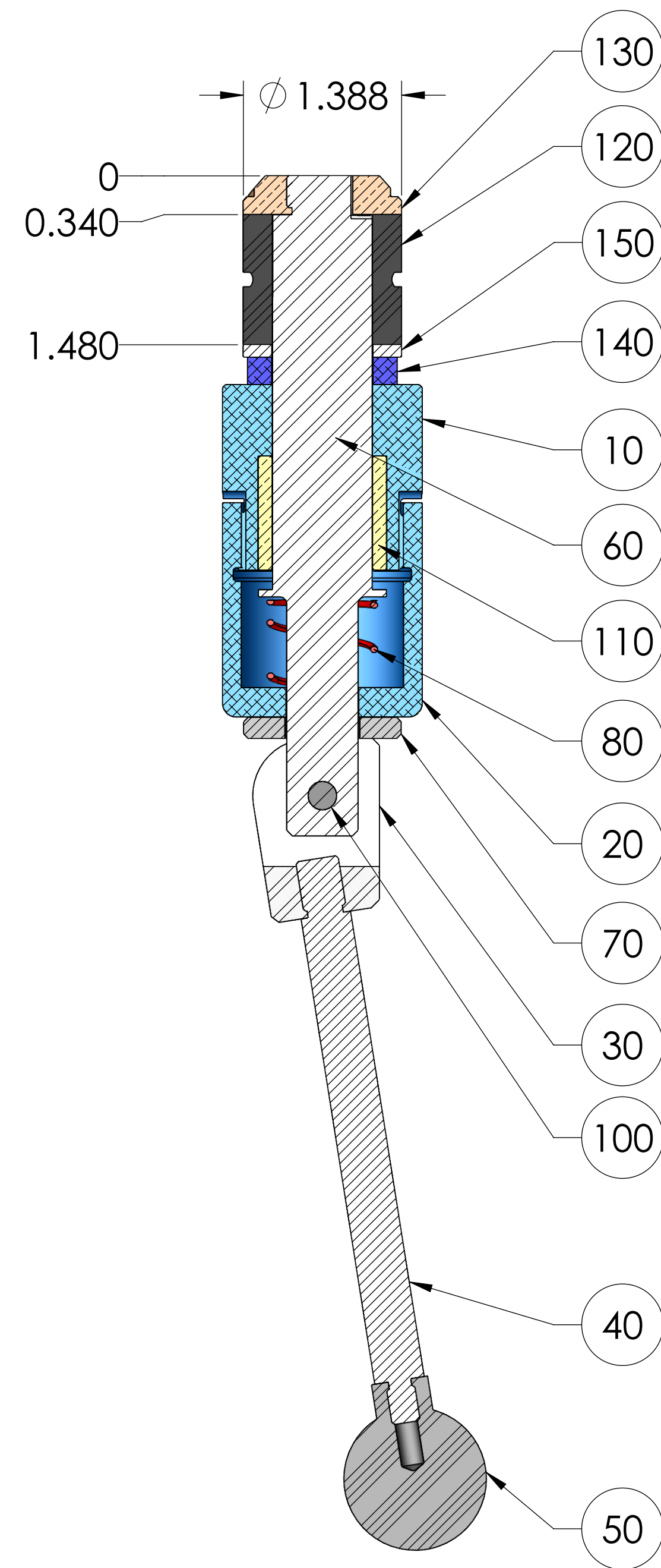
SECTION A-A
