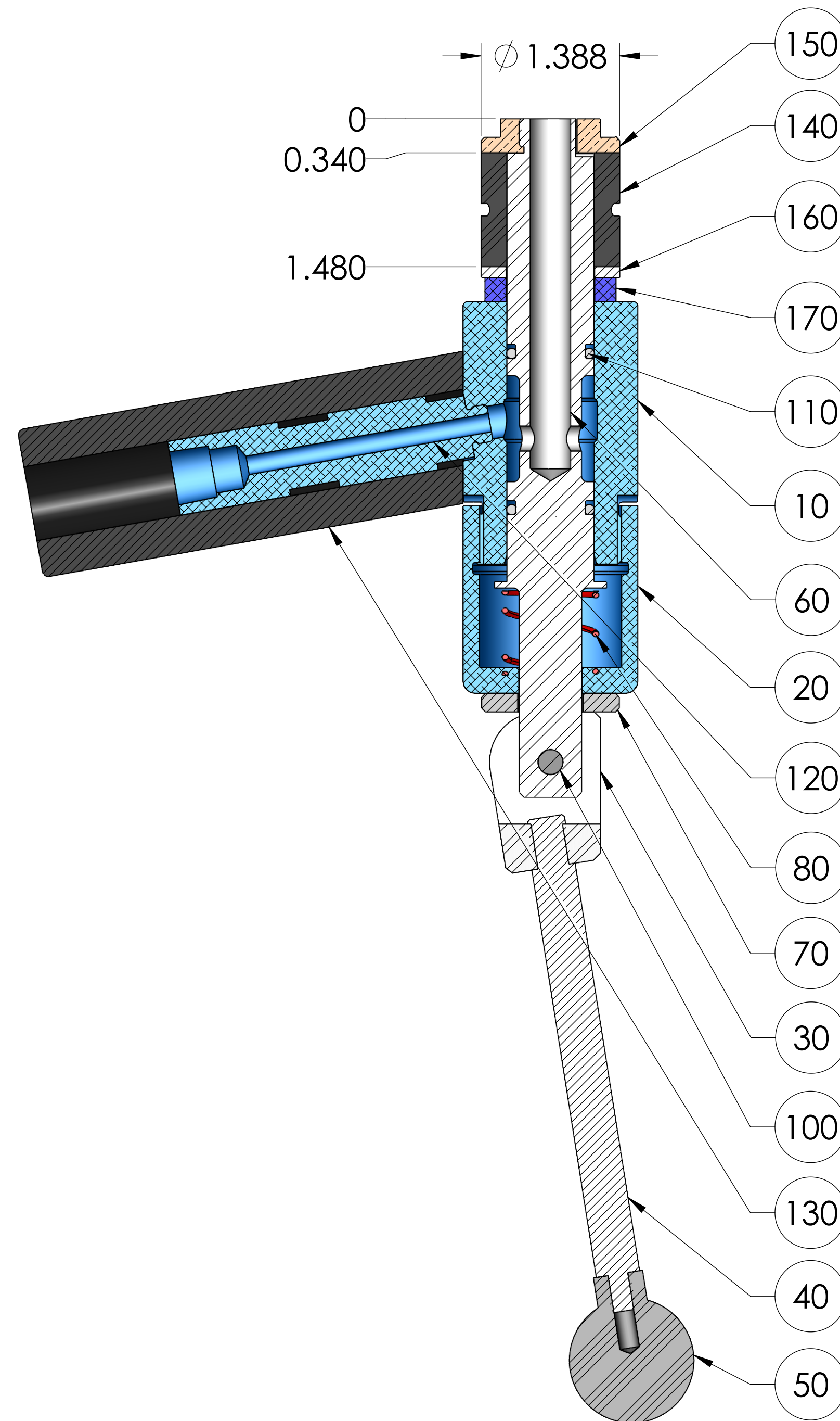
SECTION A-A
