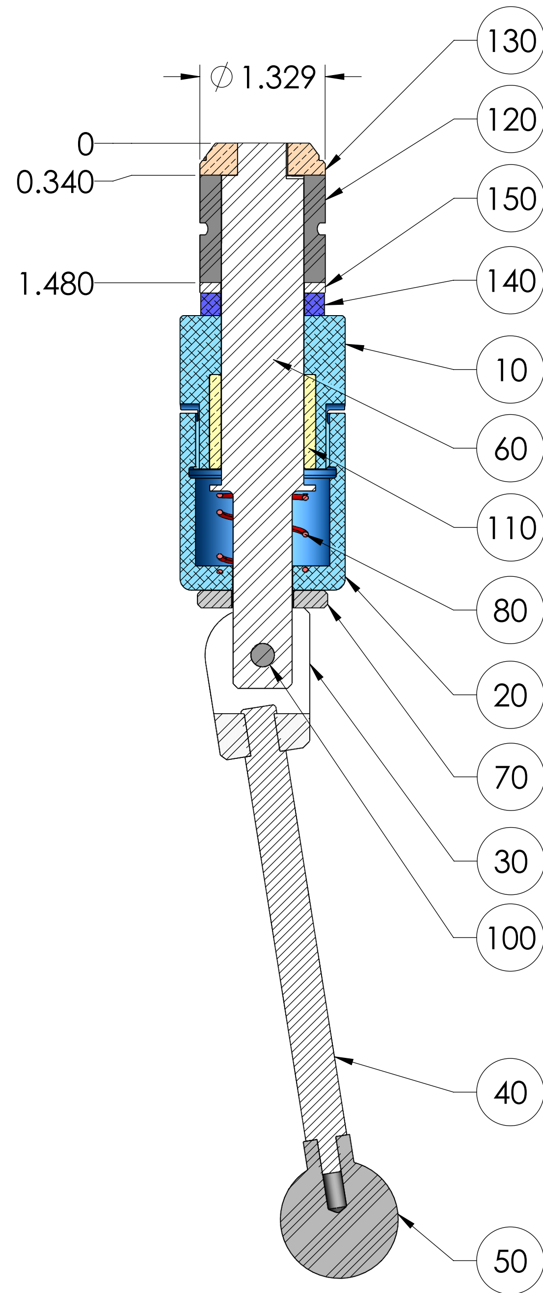
SECTION A-A
