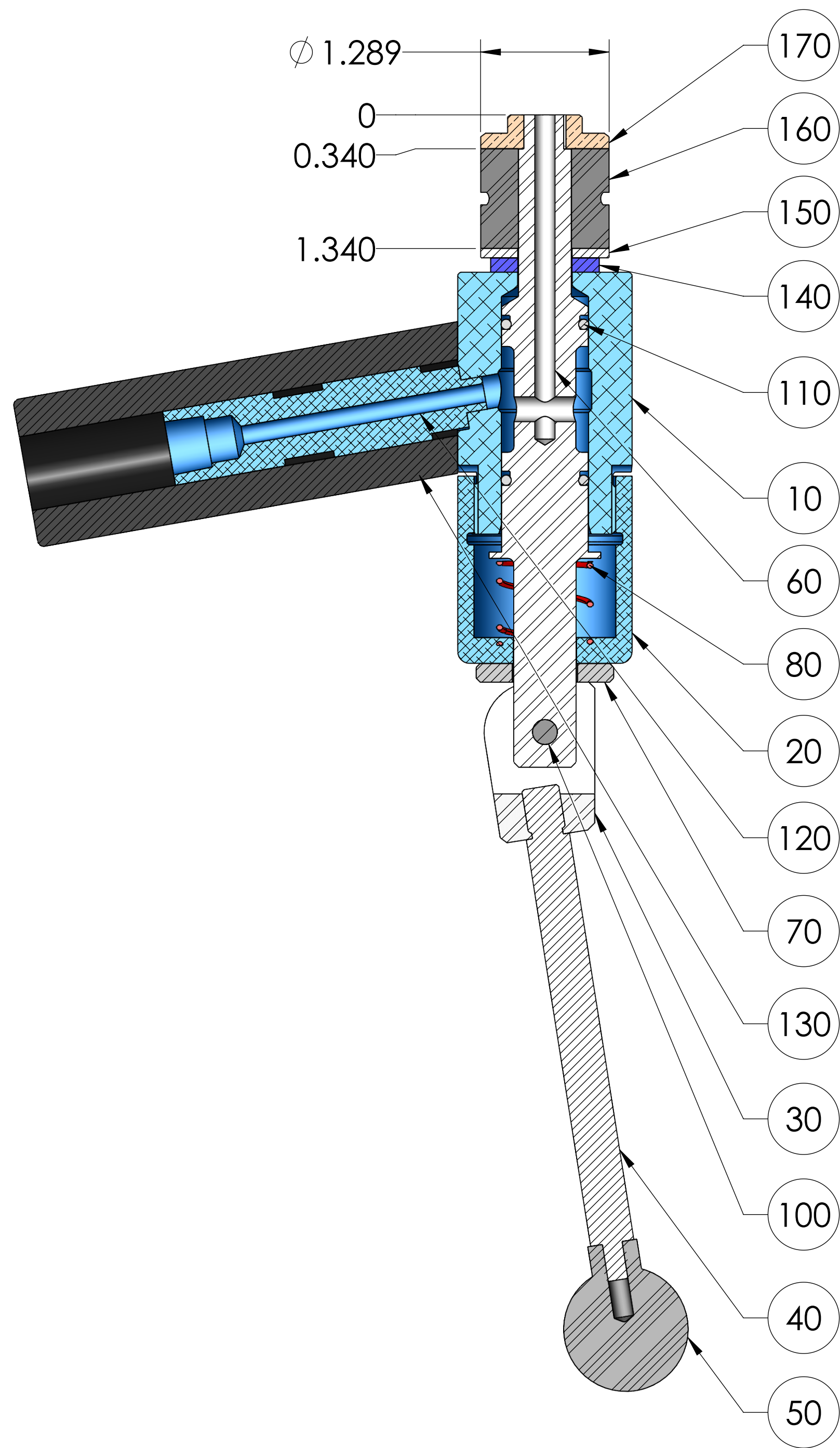
SECTION A-A
