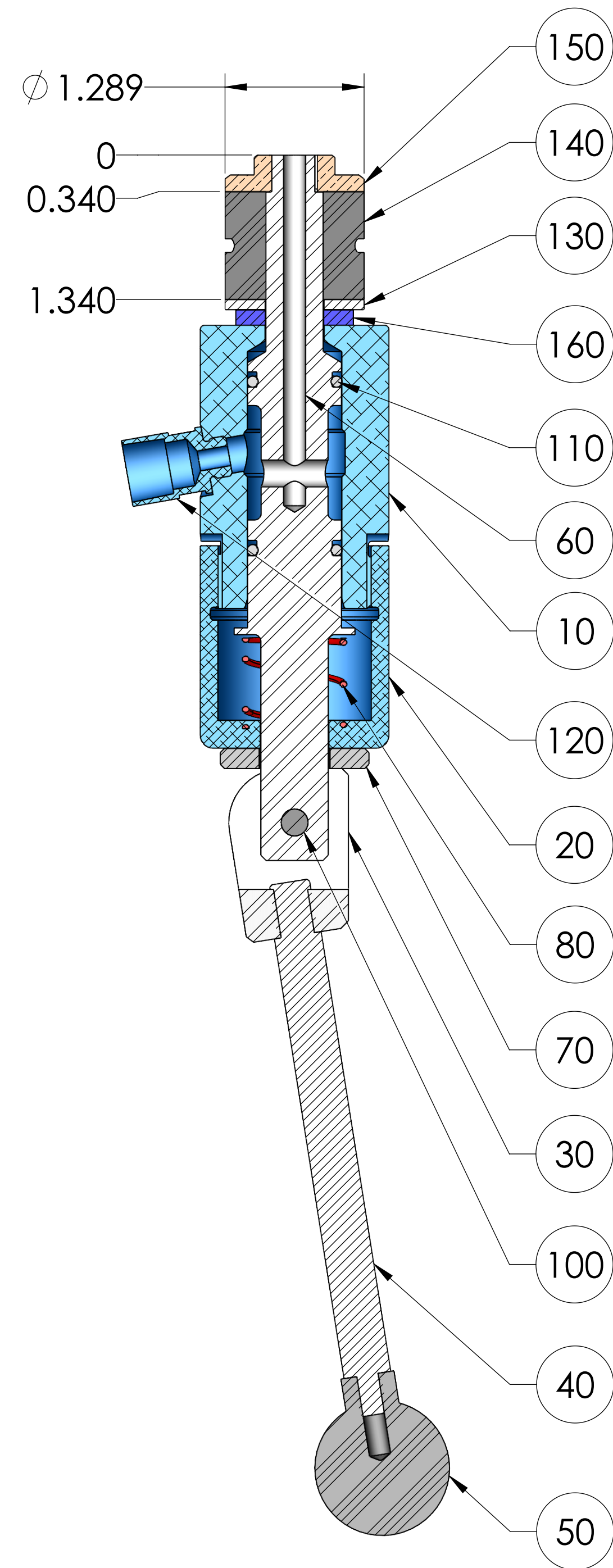
SECTION A-A
