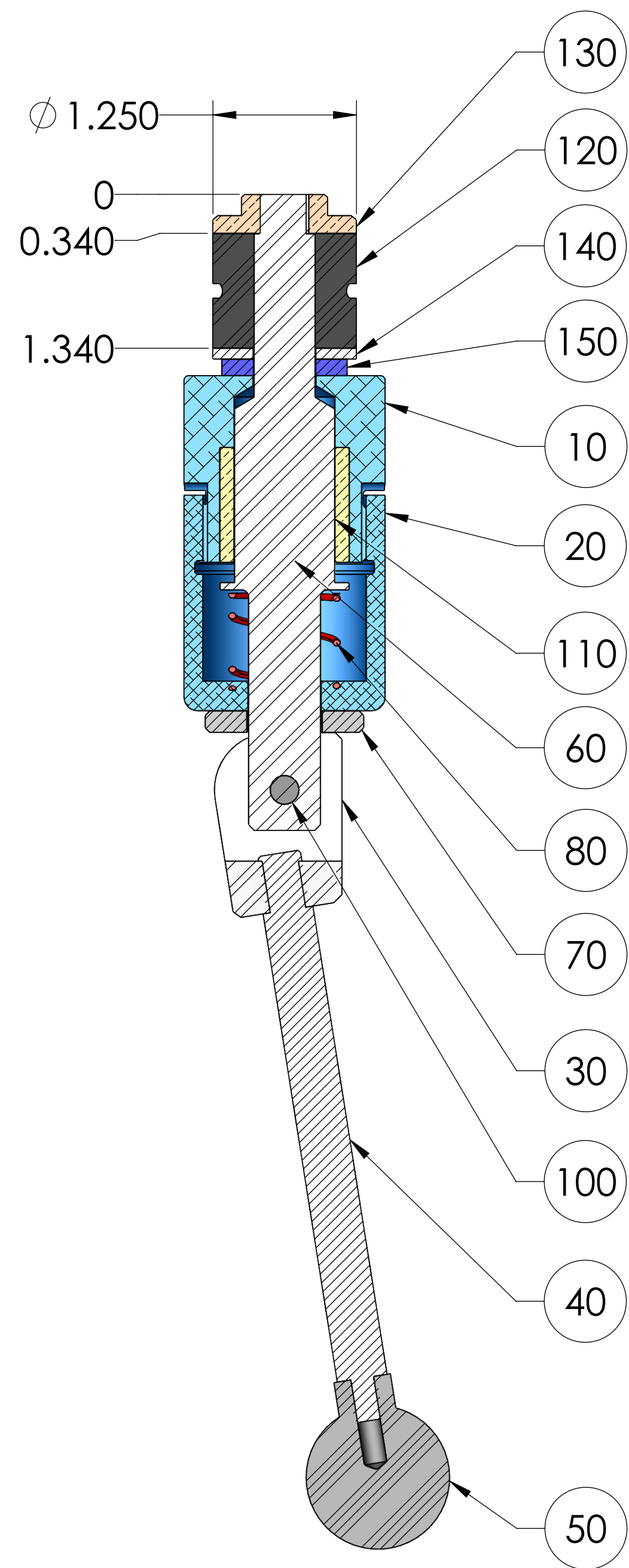
SECTION A-A
