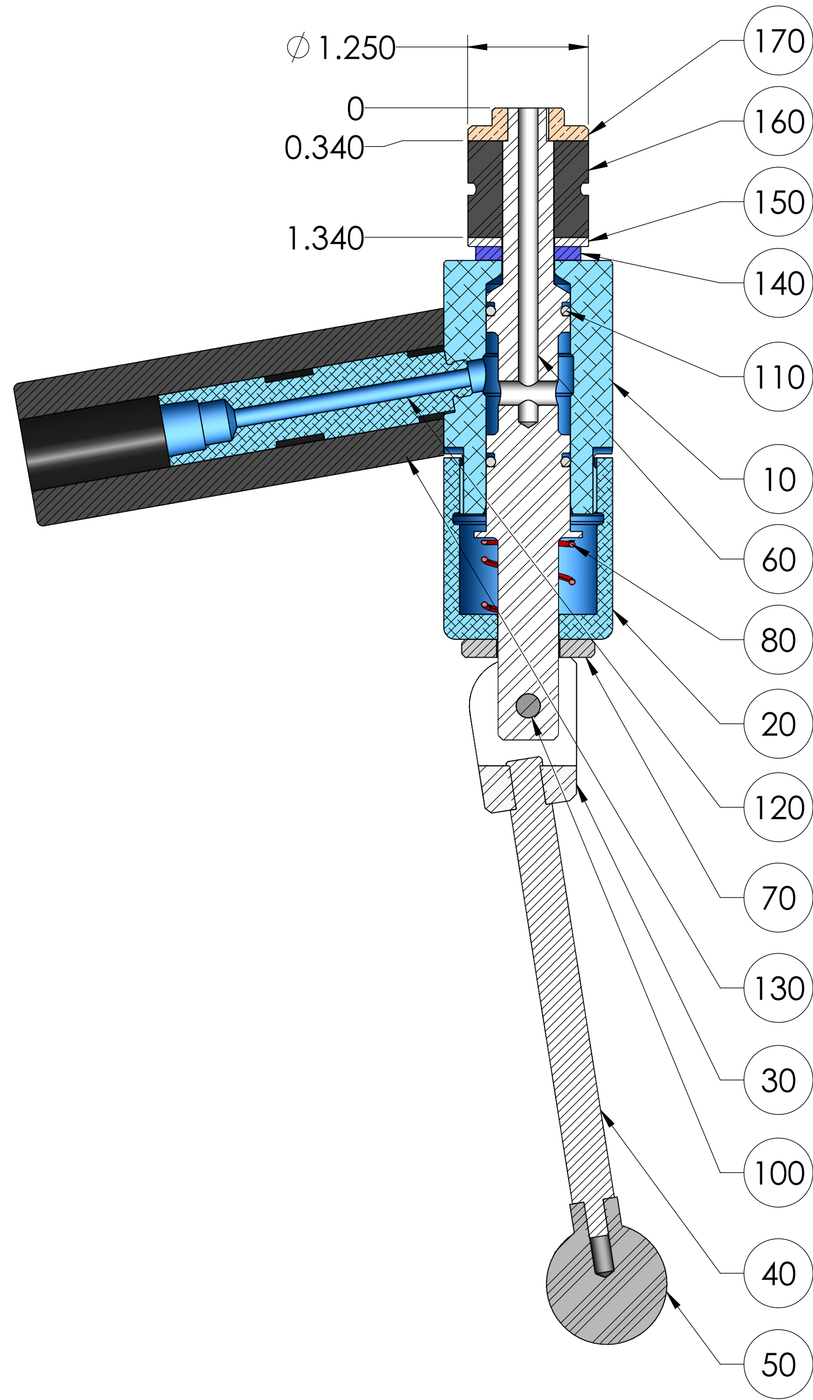
SECTION A-A
