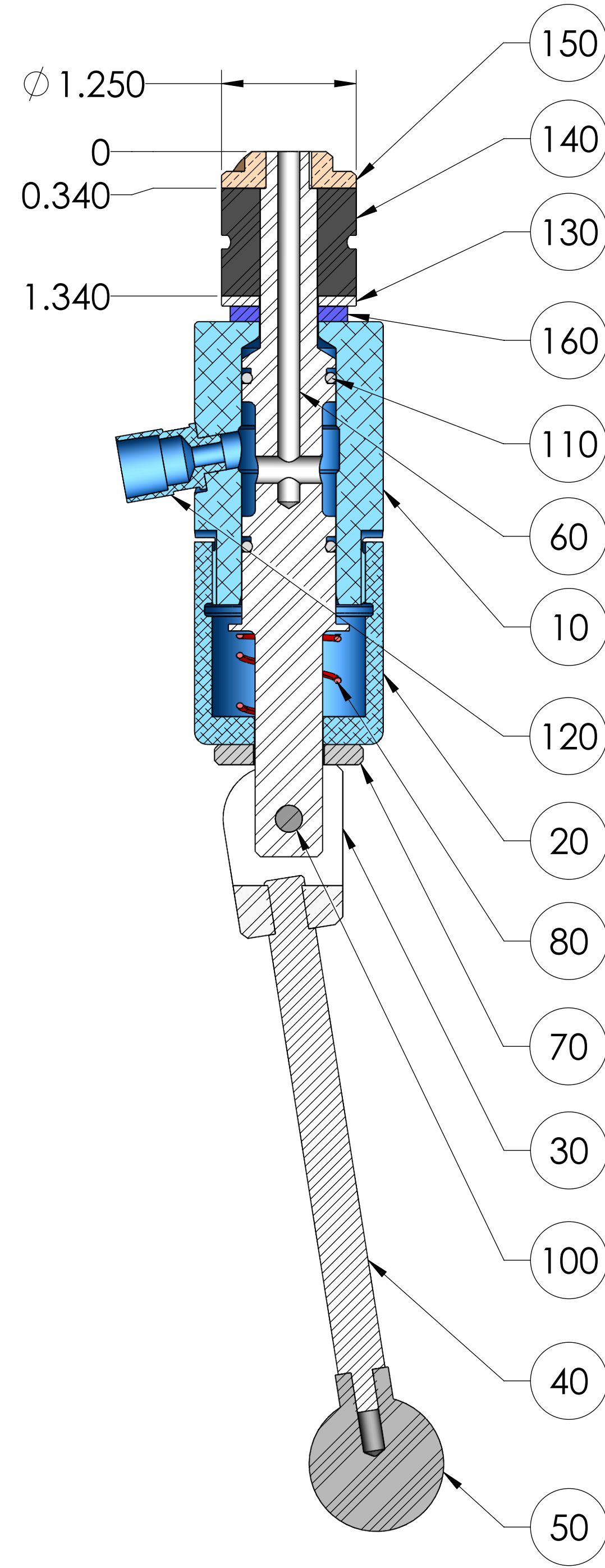
SECTION A-A
