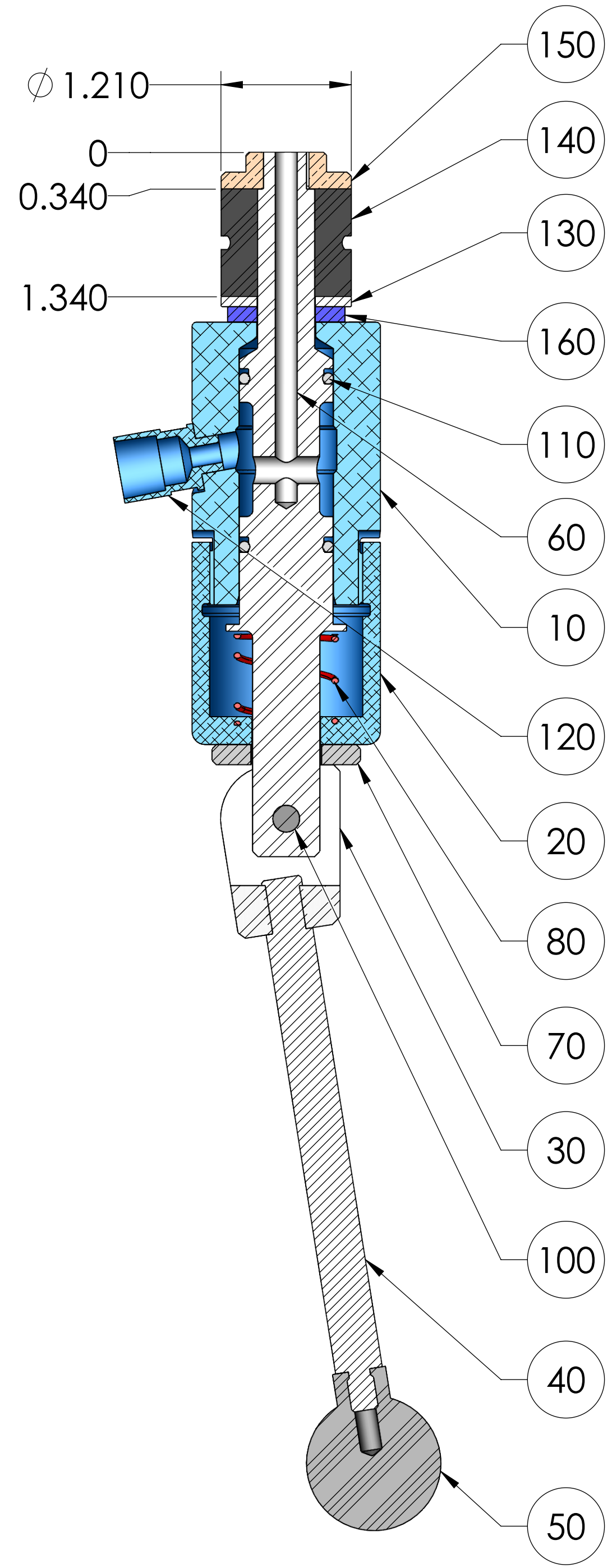
SECTION A-A
