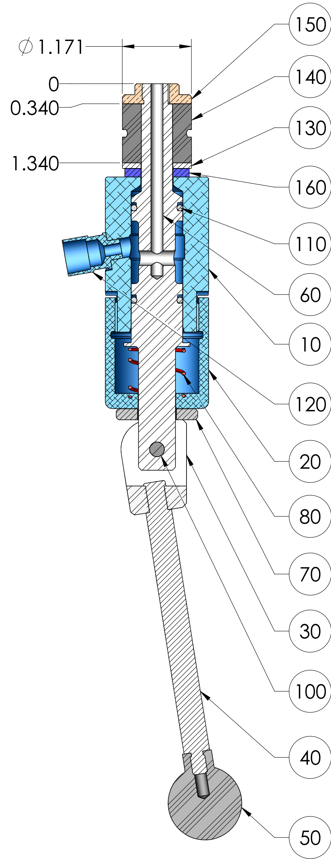
SECTION A-A
