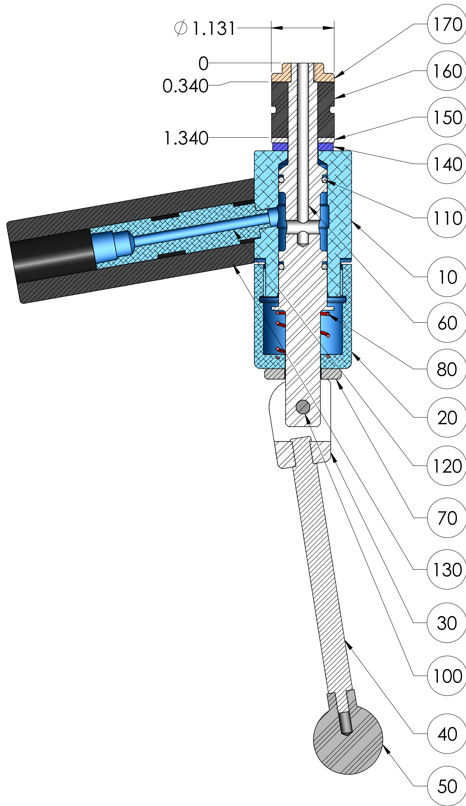
SECTION A-A
