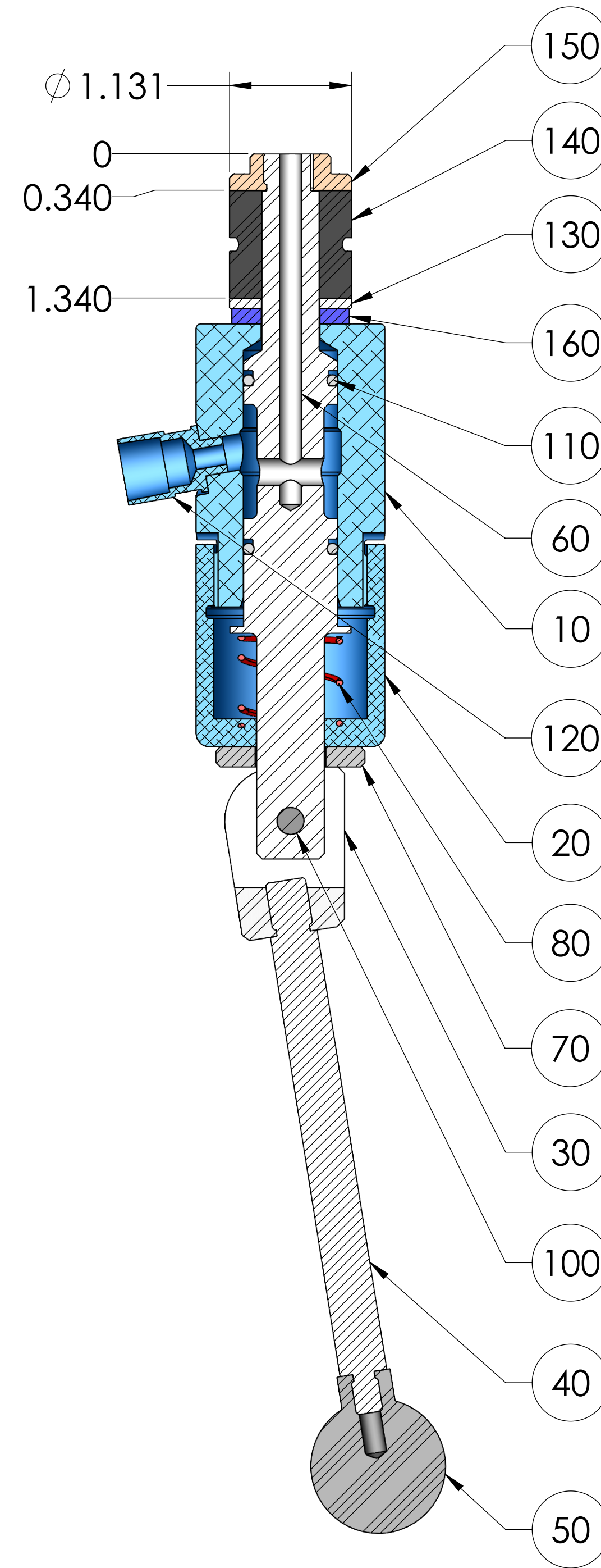
SECTION A-A
