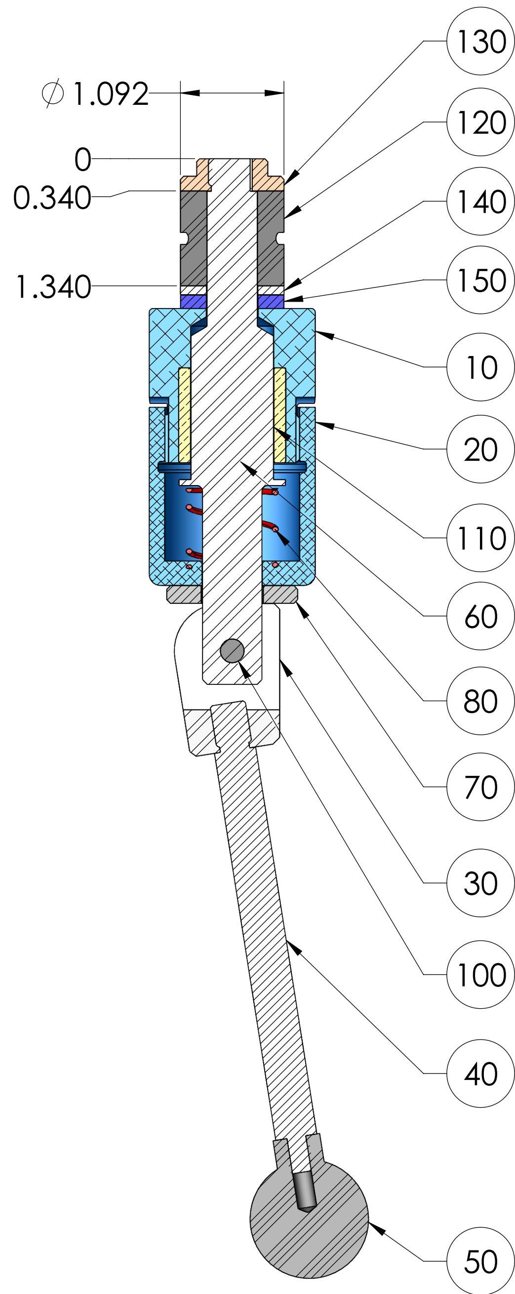
SECTION A-A
