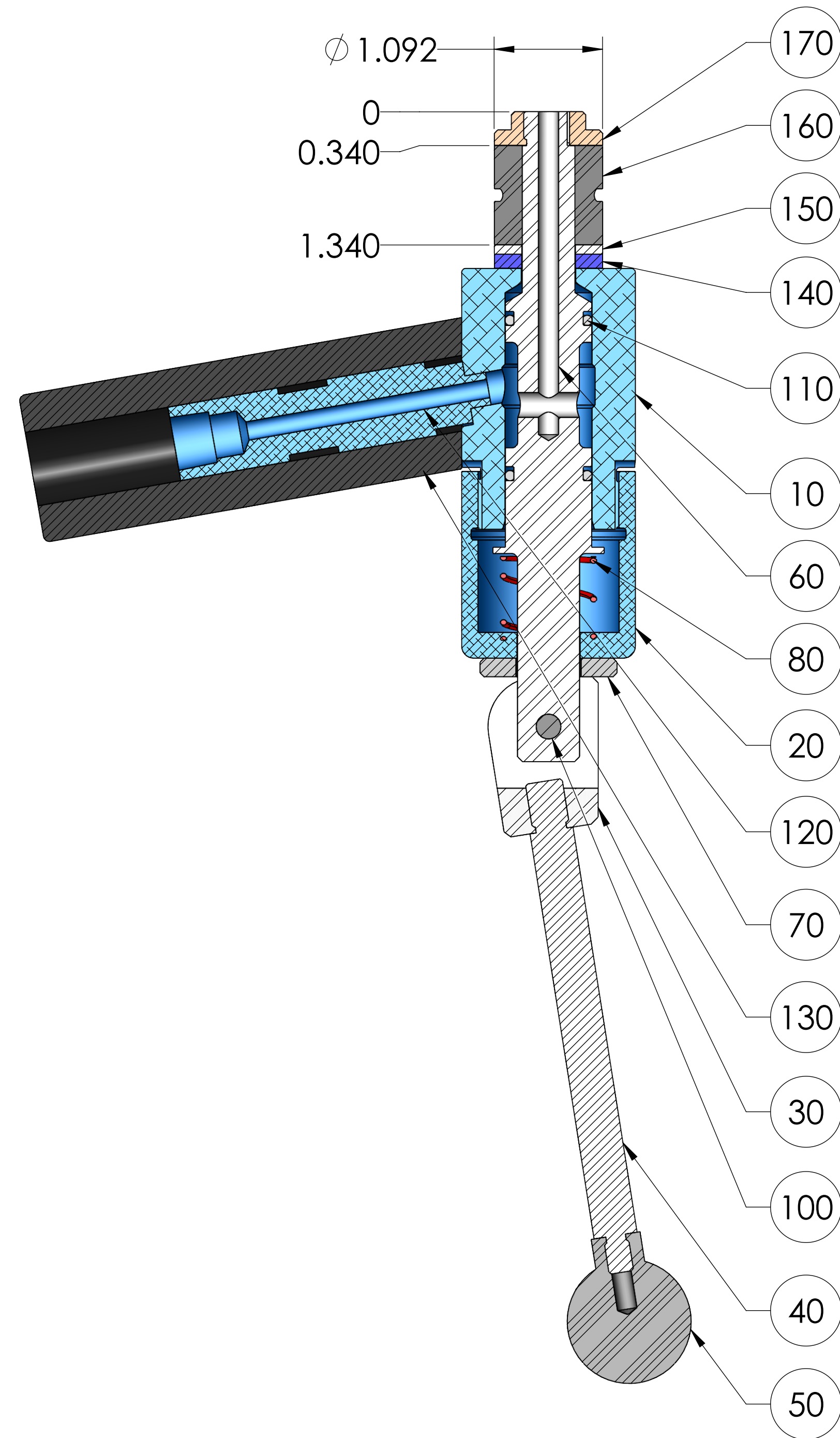
SECTION A-A
