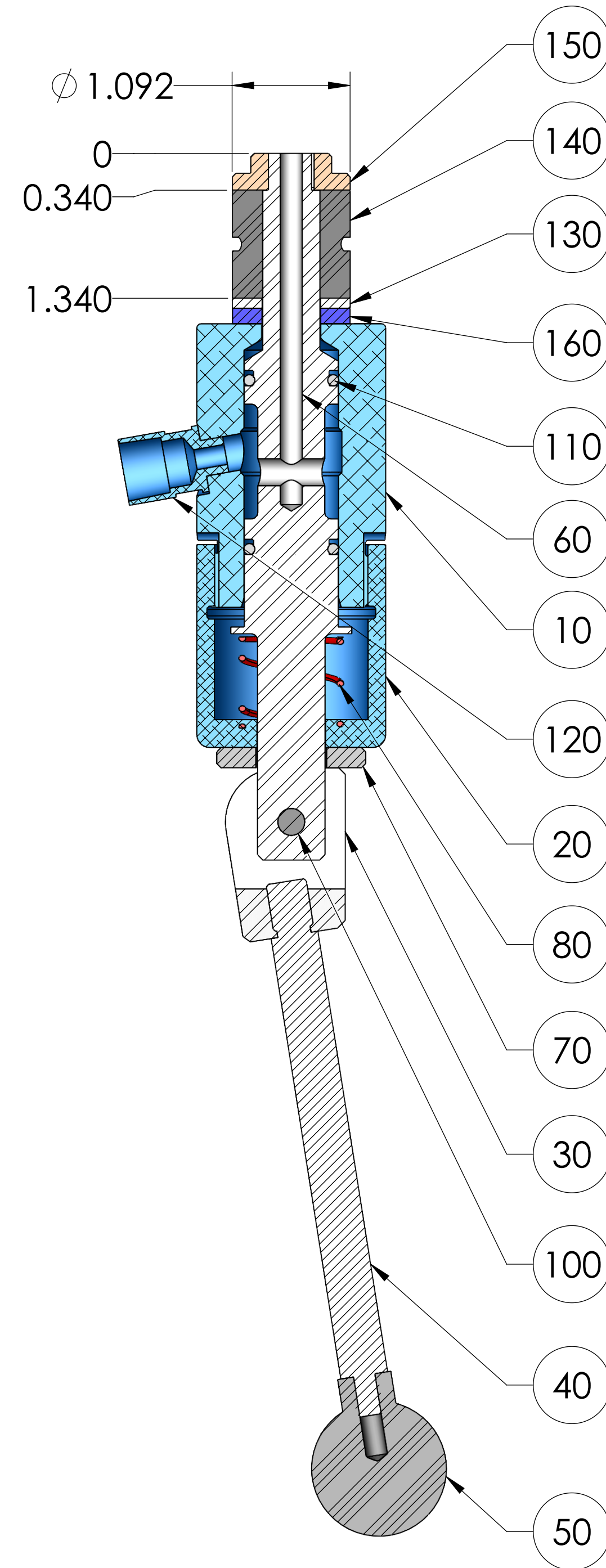
SECTION A-A
