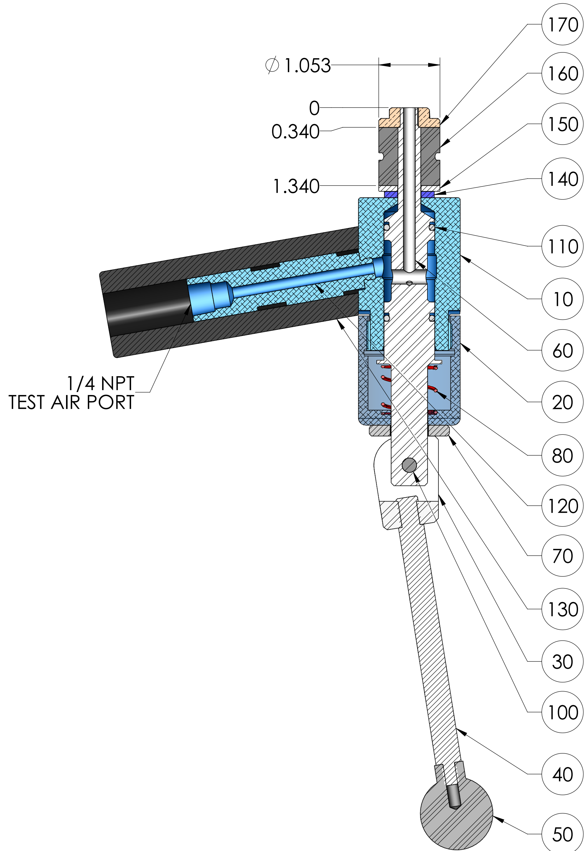
SECTION A-A
