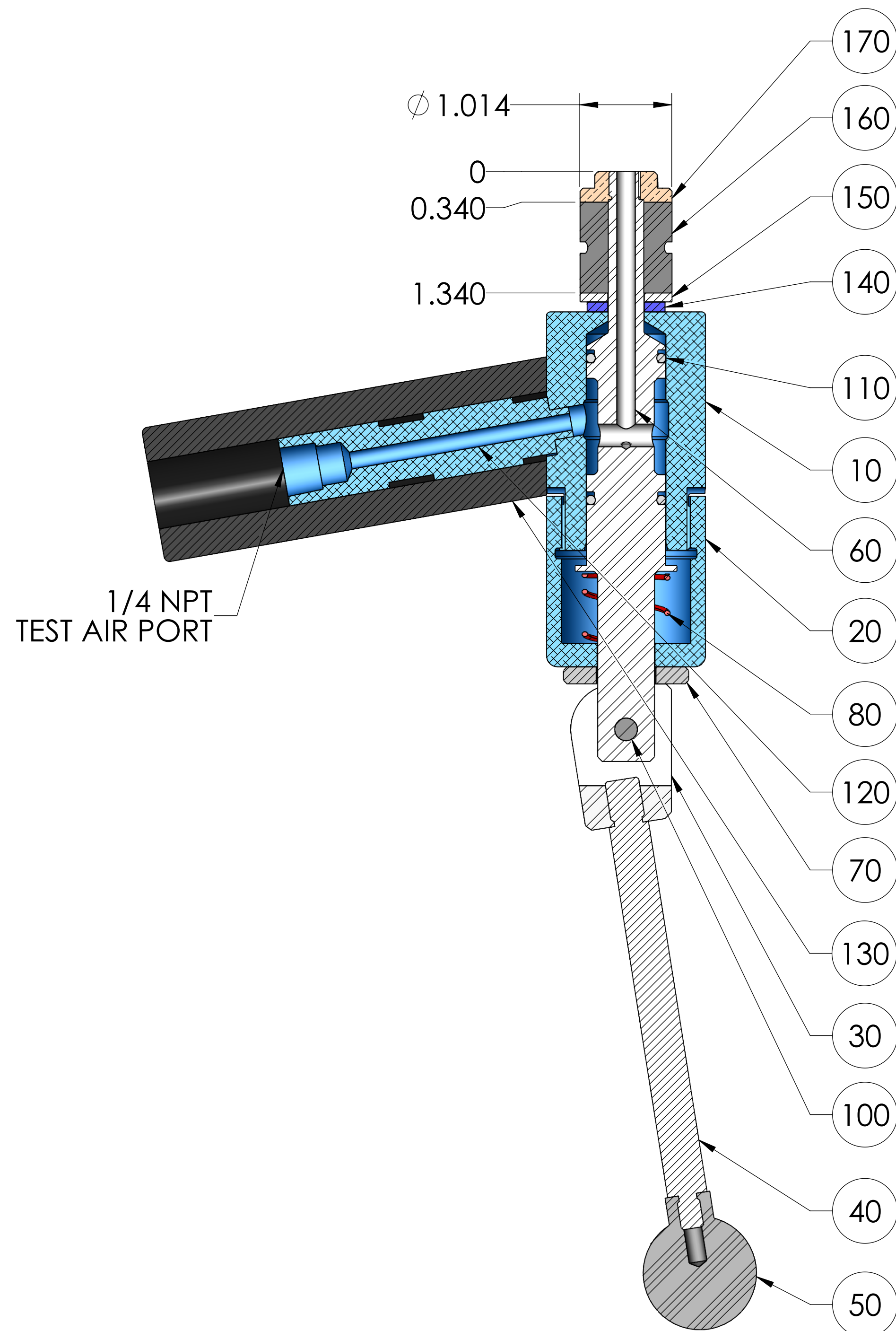
SECTION A-A
