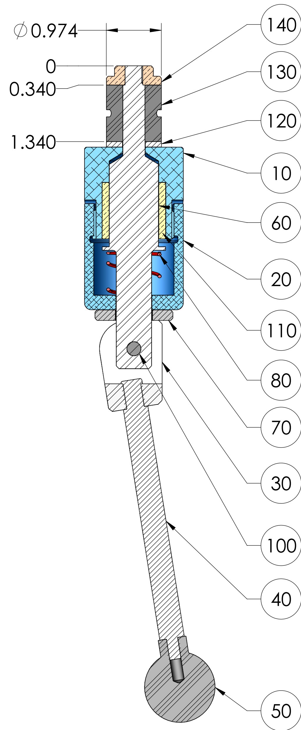
SECTION A-A
