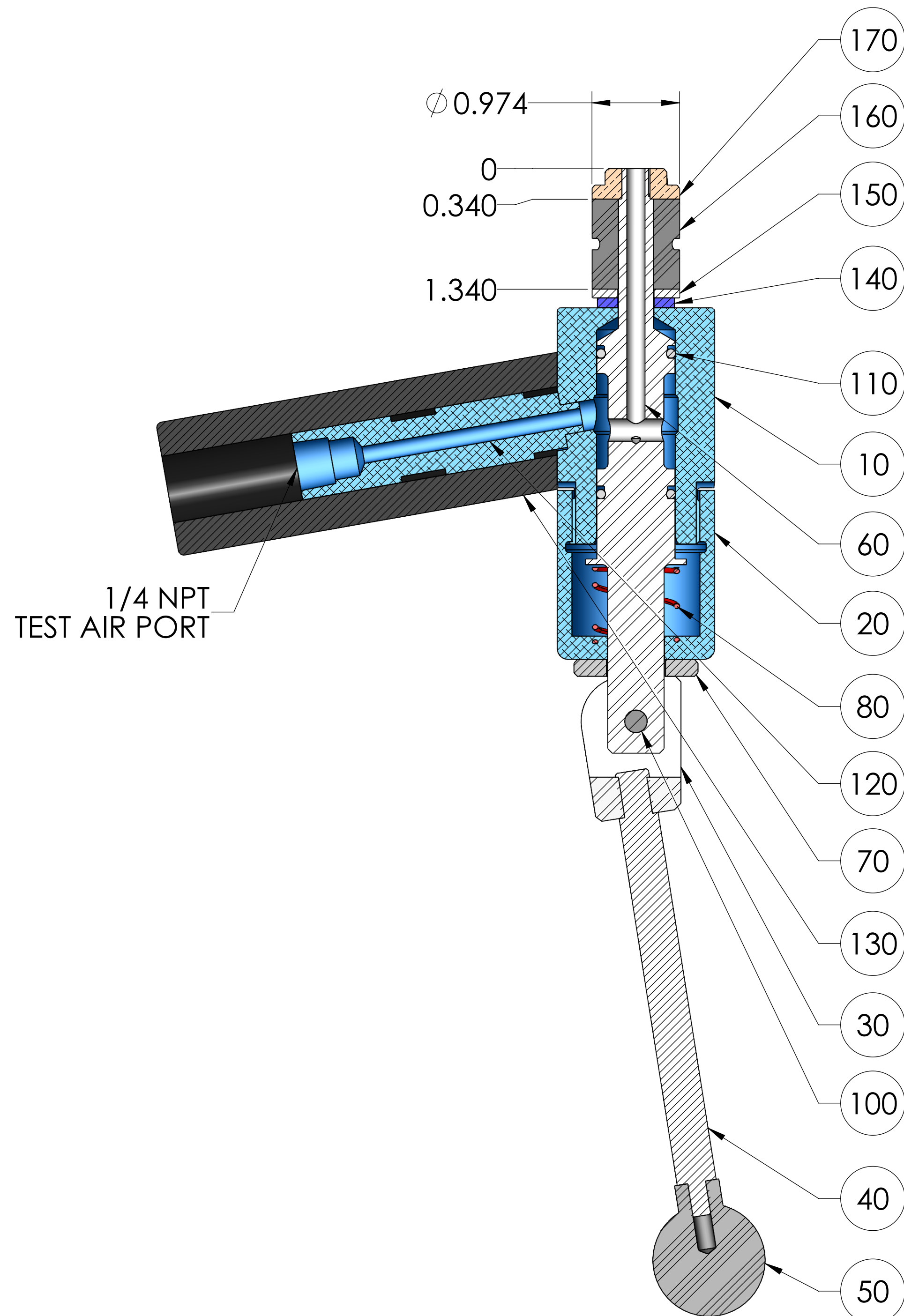
SECTION A-A
