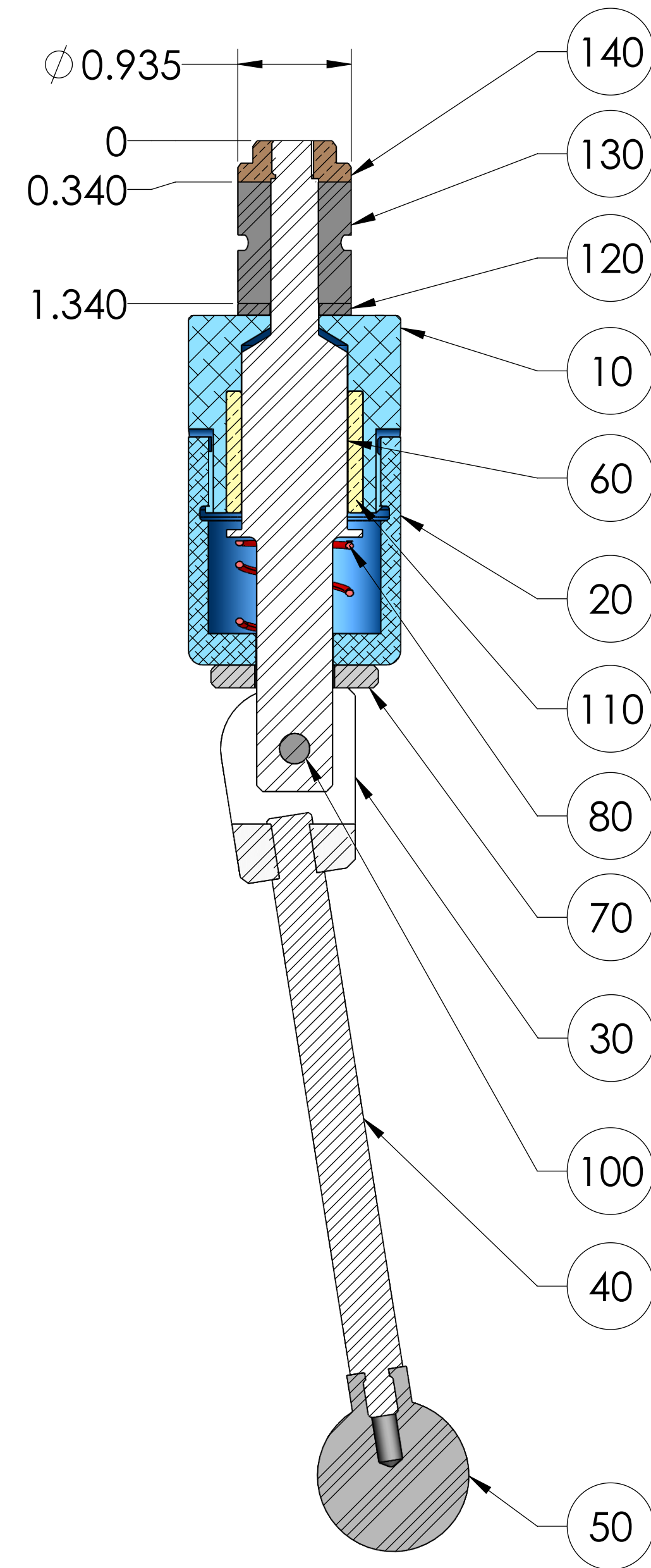
SECTION A-A
