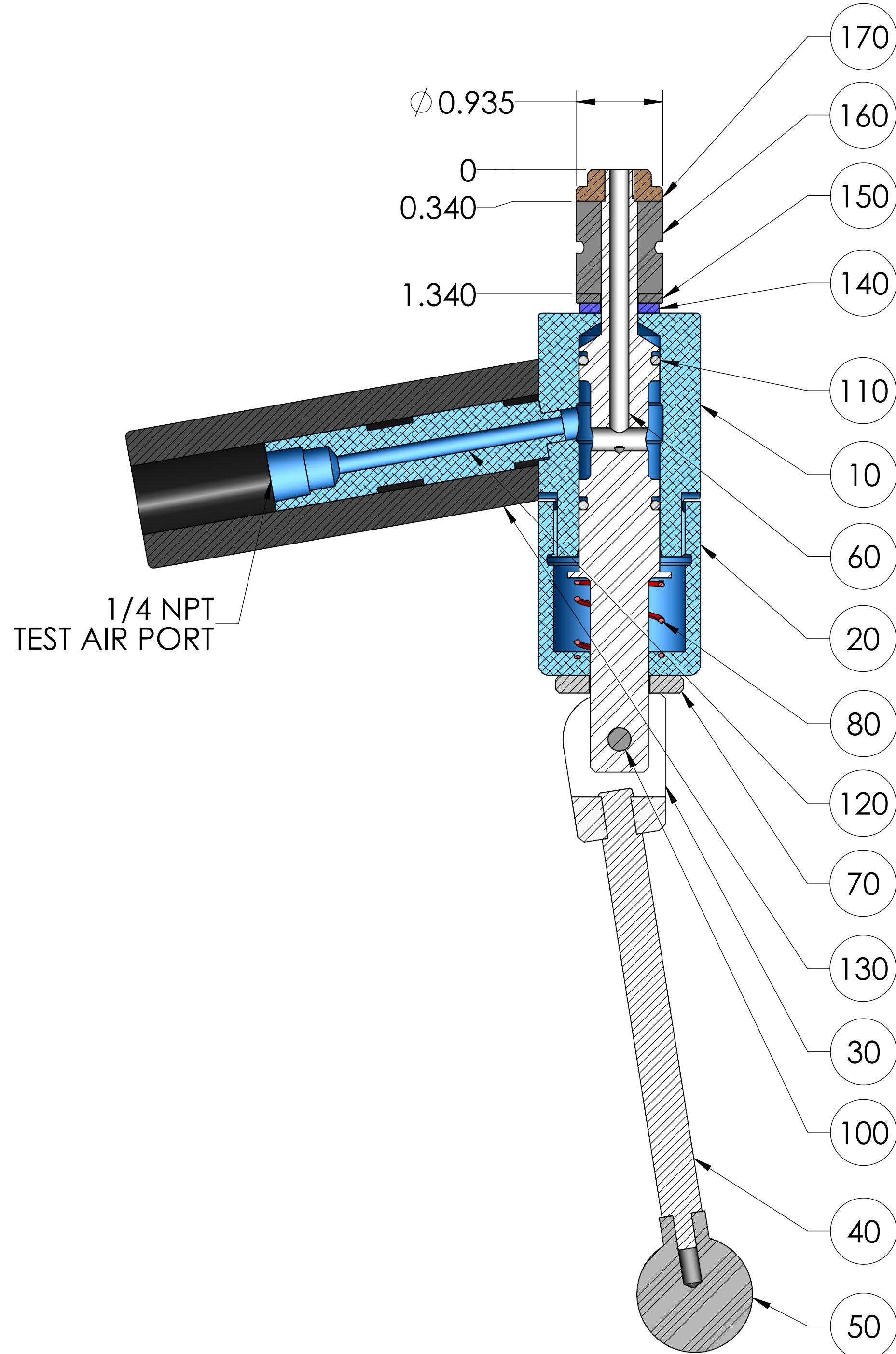
SECTION A-A
