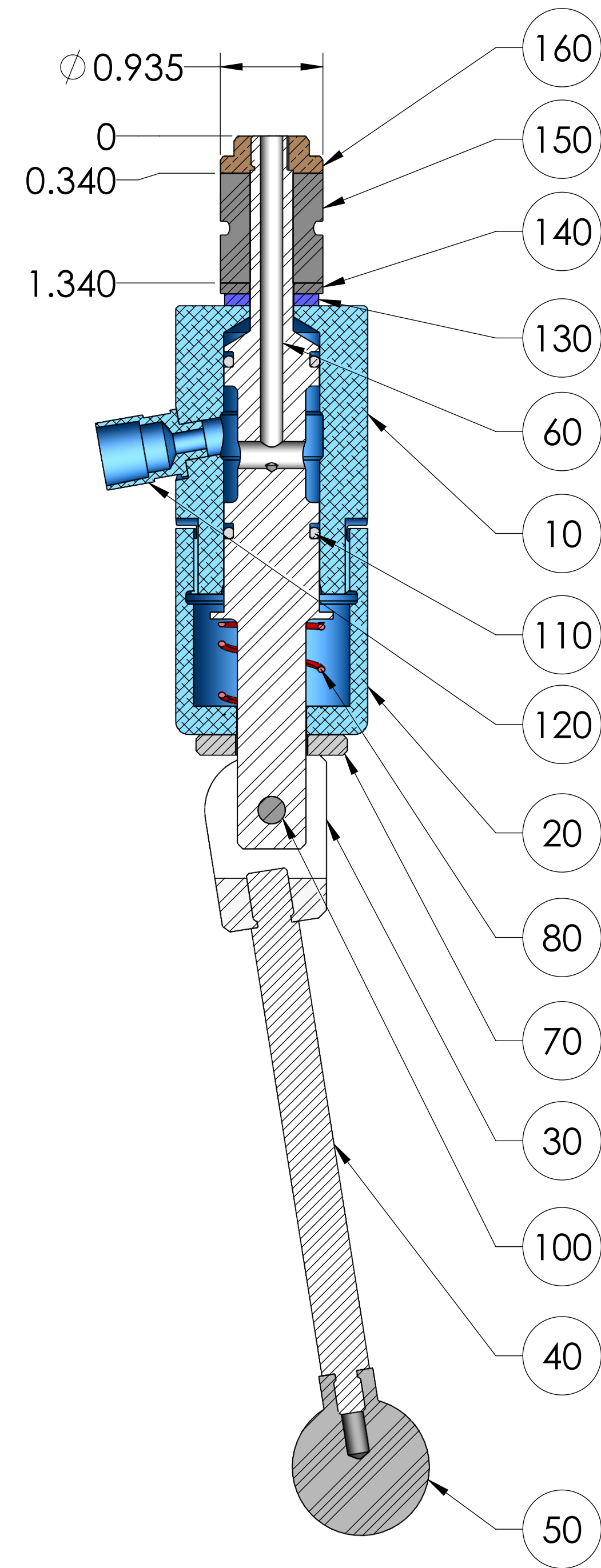
SECTION A-A
