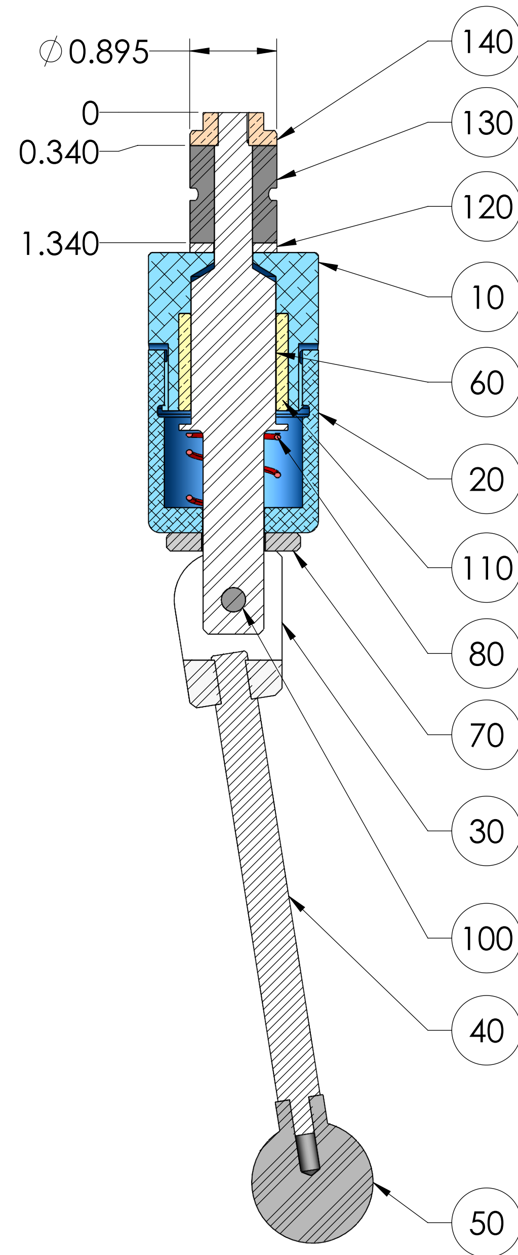
SECTION A-A
