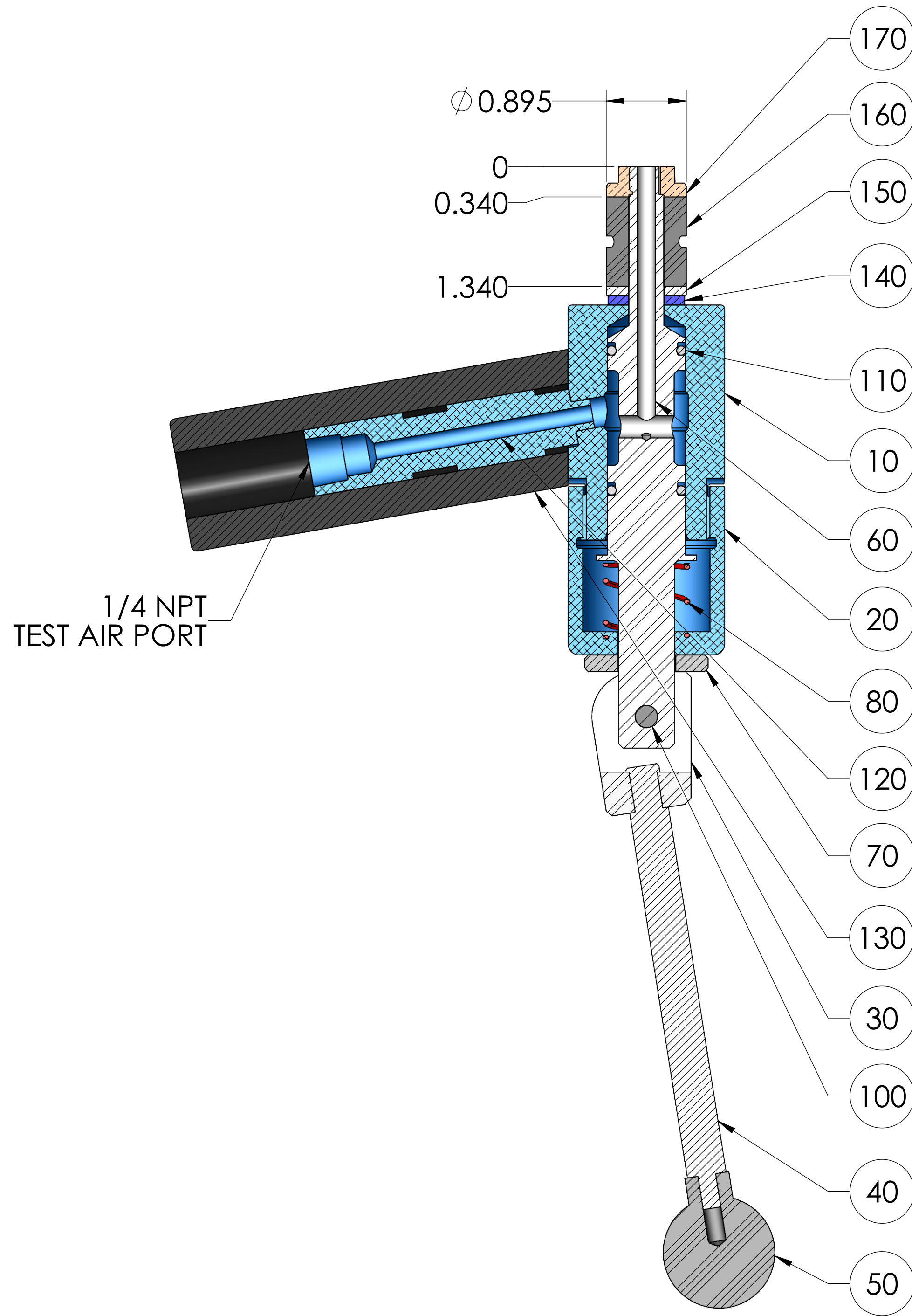
SECTION A-A
