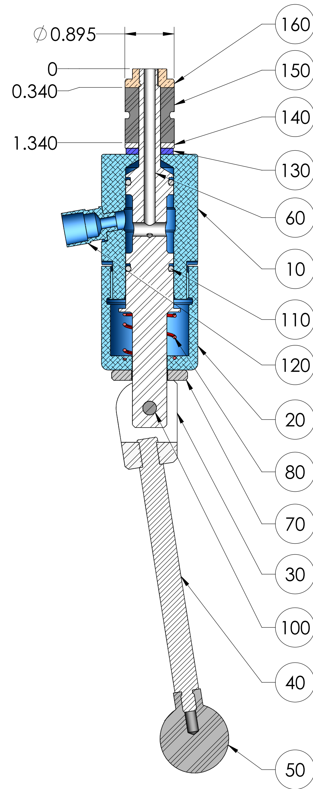
SECTION A-A
