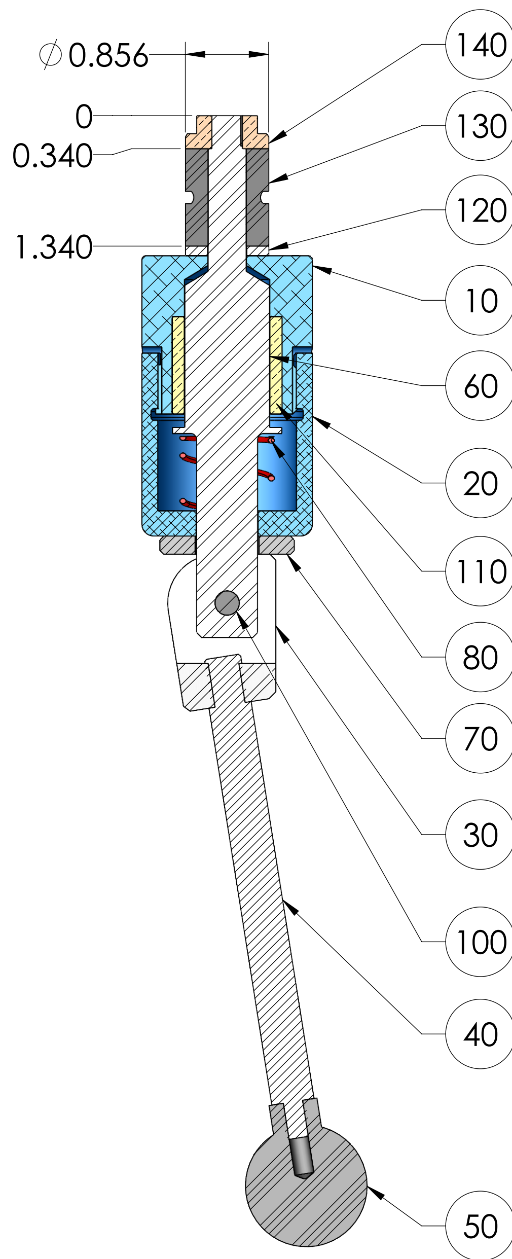
SECTION A-A
