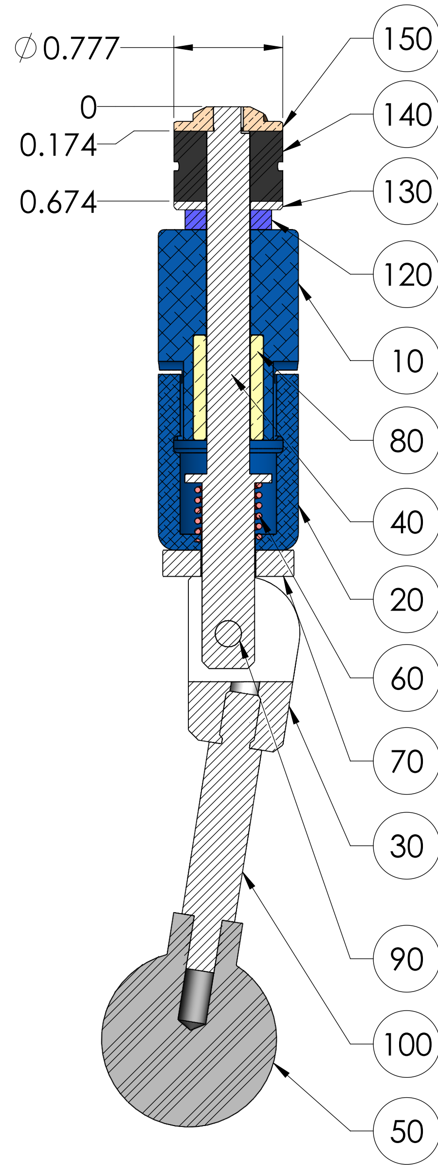
SECTION A-A SCALE 1.5 : 1
