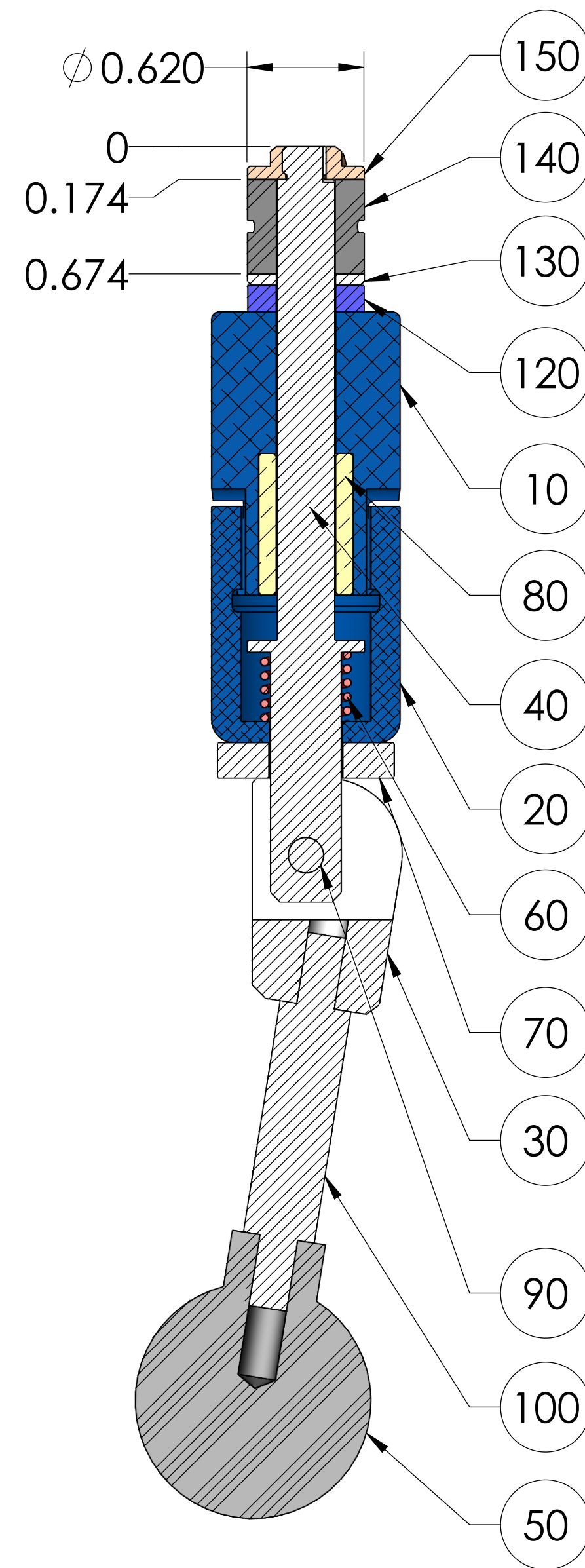
SECTION A-A SCALE 1.5 : 1
