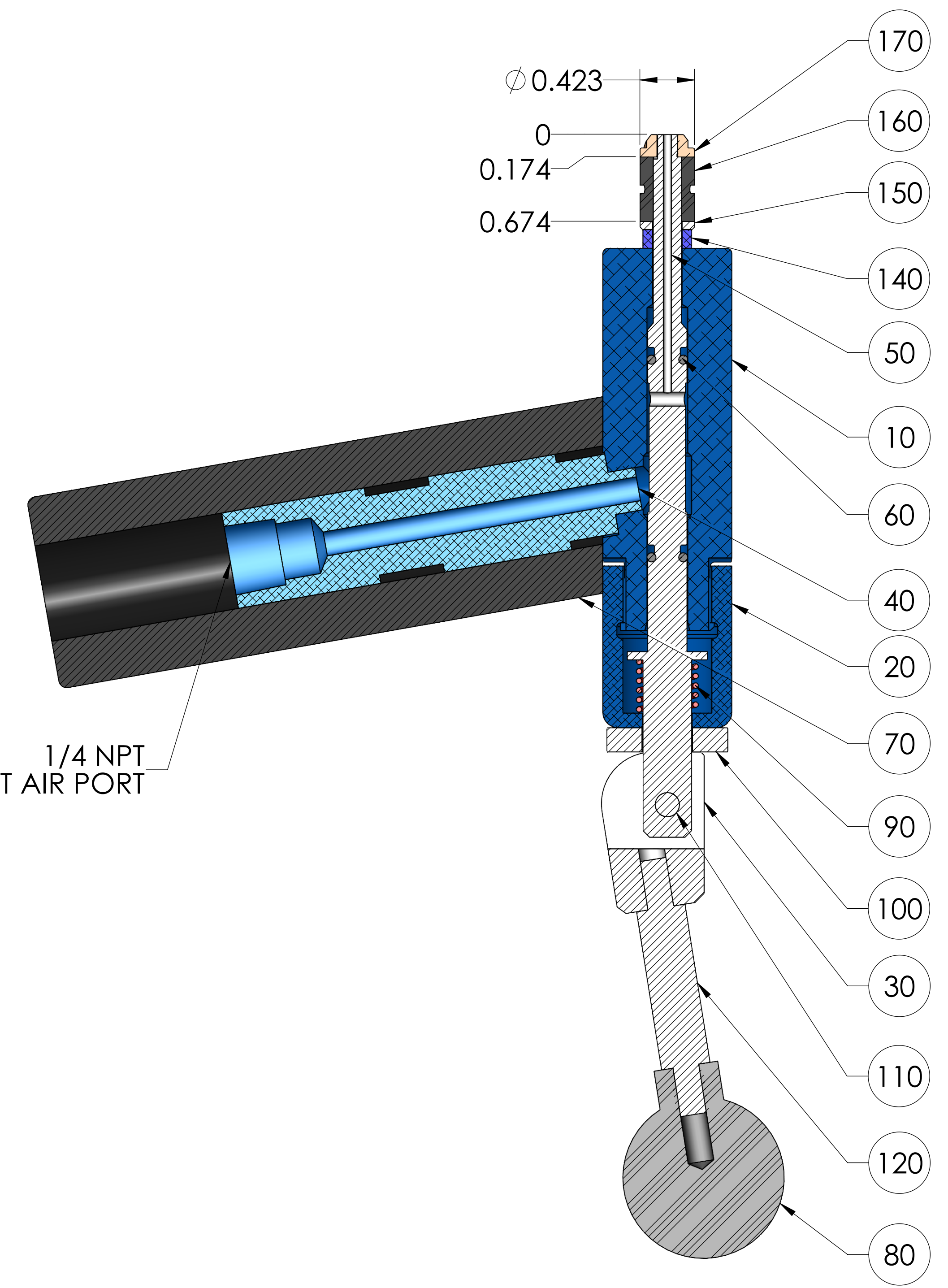
SECTION A-A SCALE 1.5 : 1
