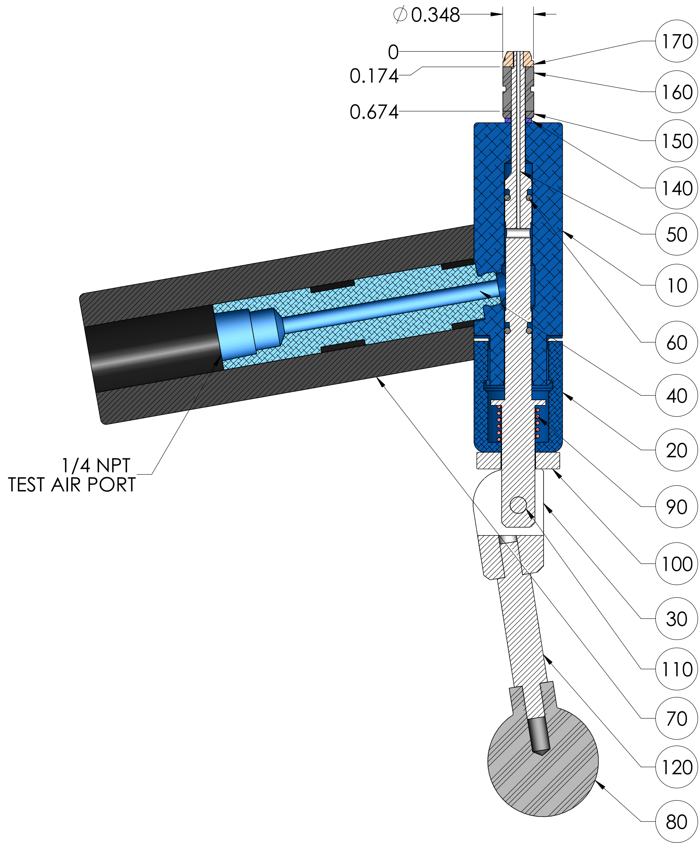
SECTION A-A SCALE 1.5 : 1
