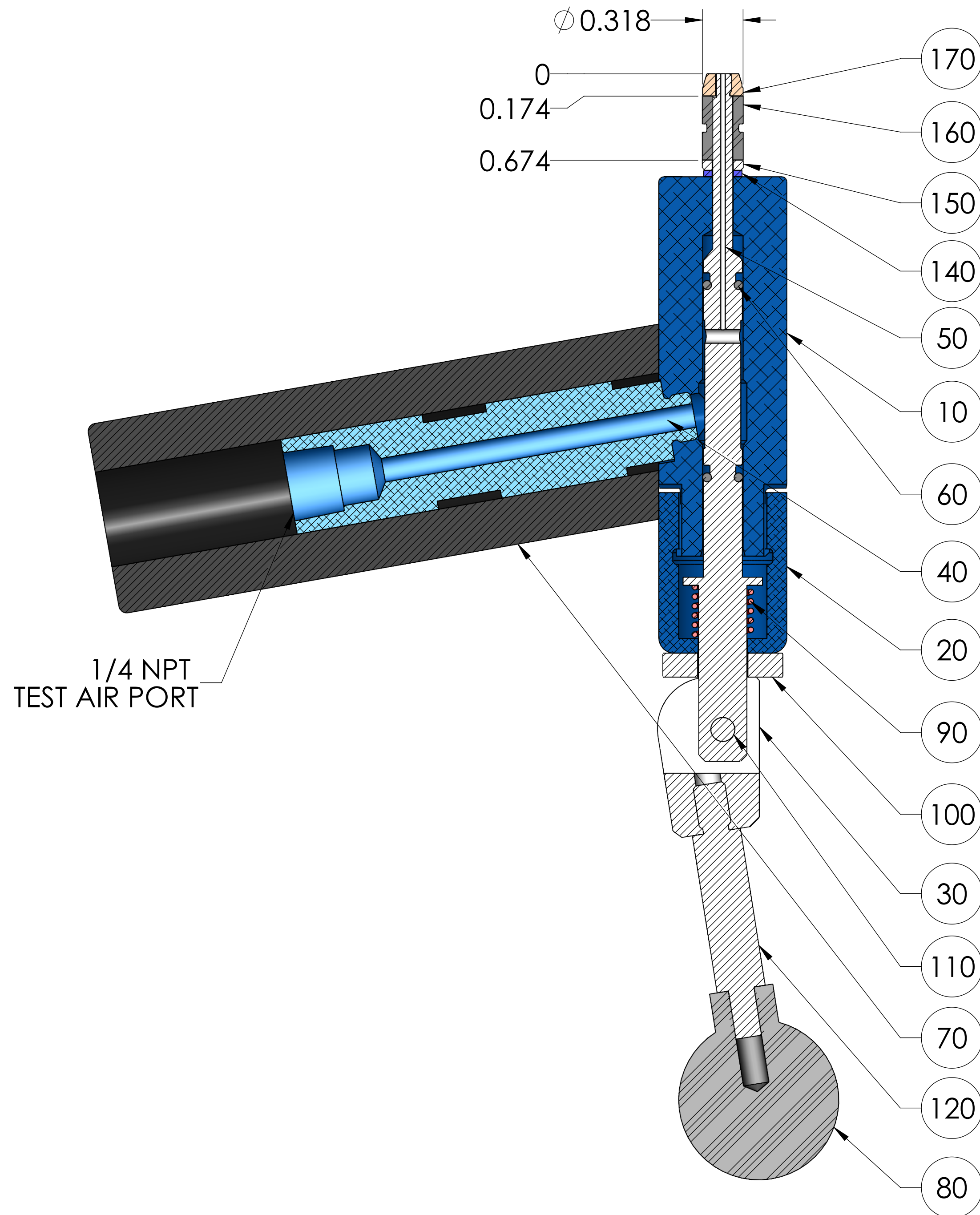
SECTION A-A SCALE 1.5 : 1
