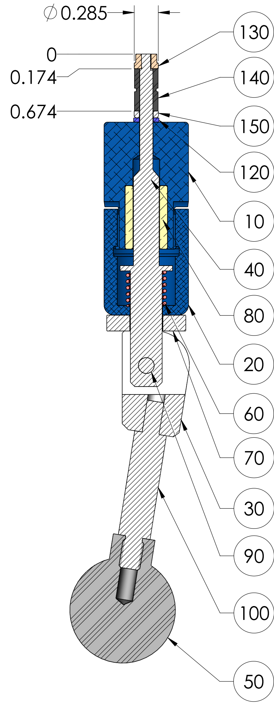
SECTION A-A SCALE 1.5 : 1
